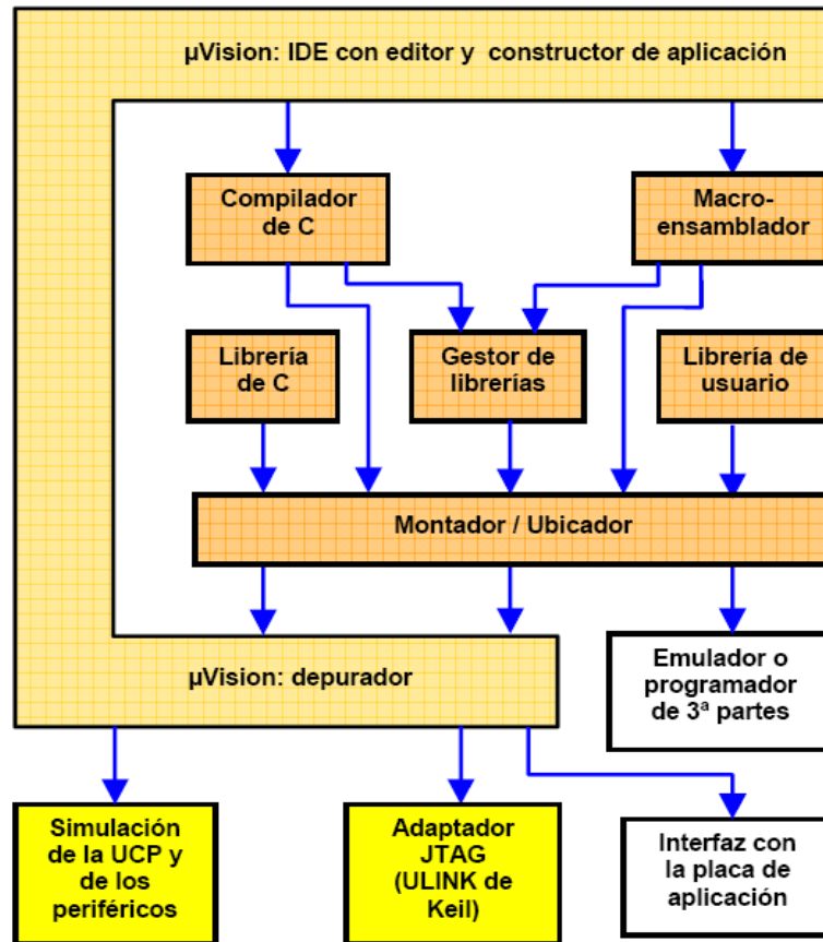
Figura 1. Componentes del entorno de desarrollo Keil \mu Vision ® .
