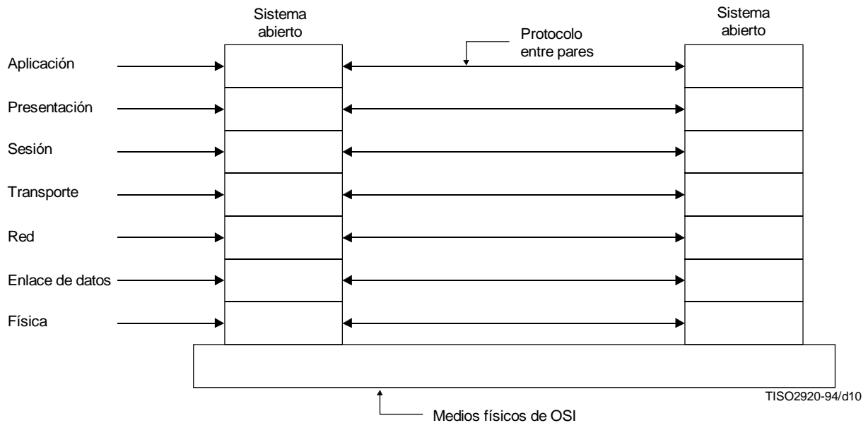
Figura 11 – Modelo de referencia de siete capas y protocolos entre pares
