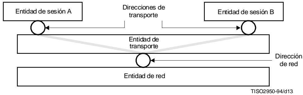
Figura 14 – Asociación de una dirección de red con varias direcciones de transporte
