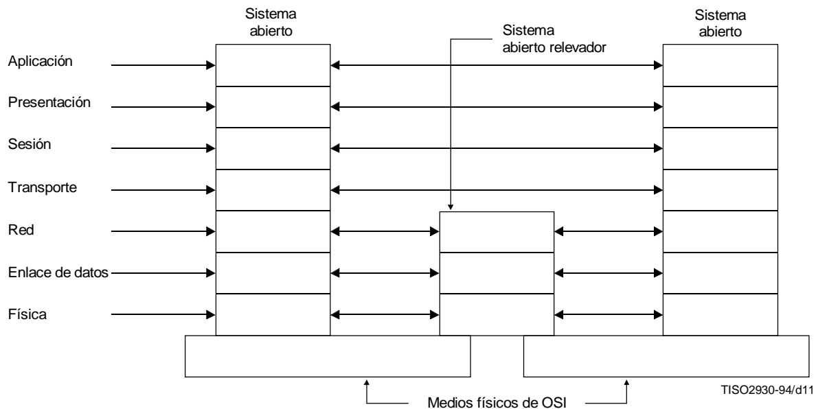
Figura 12 – Comunicaciones con la intervención de sistemas abiertos relevadores
