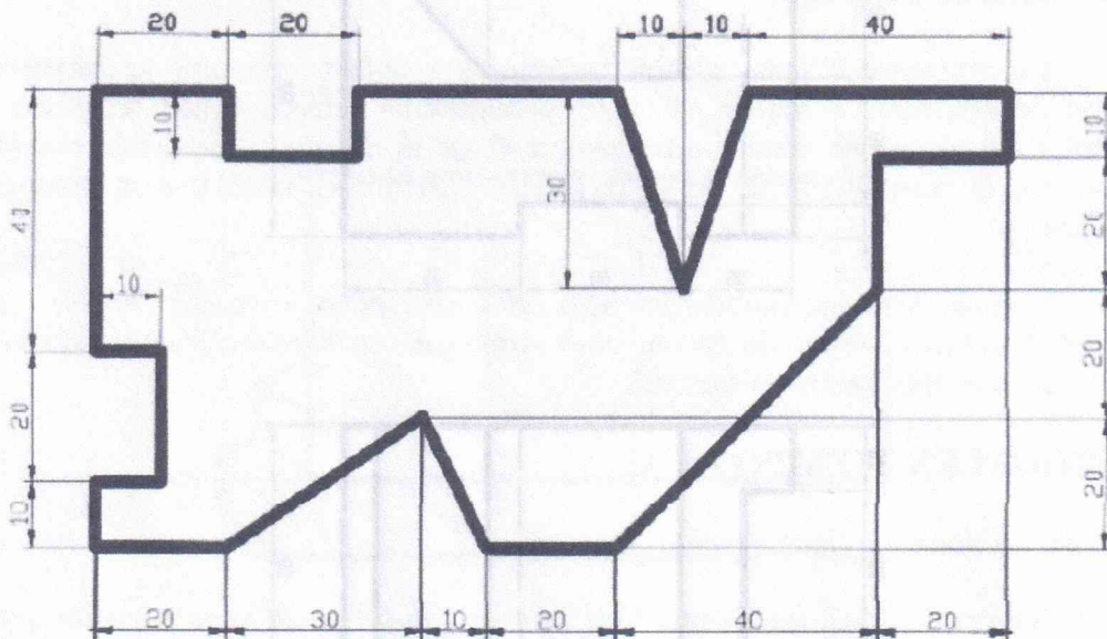
Figura 7.2. Planta para el uso del comando elev.
