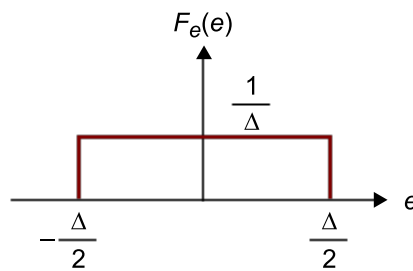
Figura 5. Función de densidad de probabilidad del error de cuantificación
