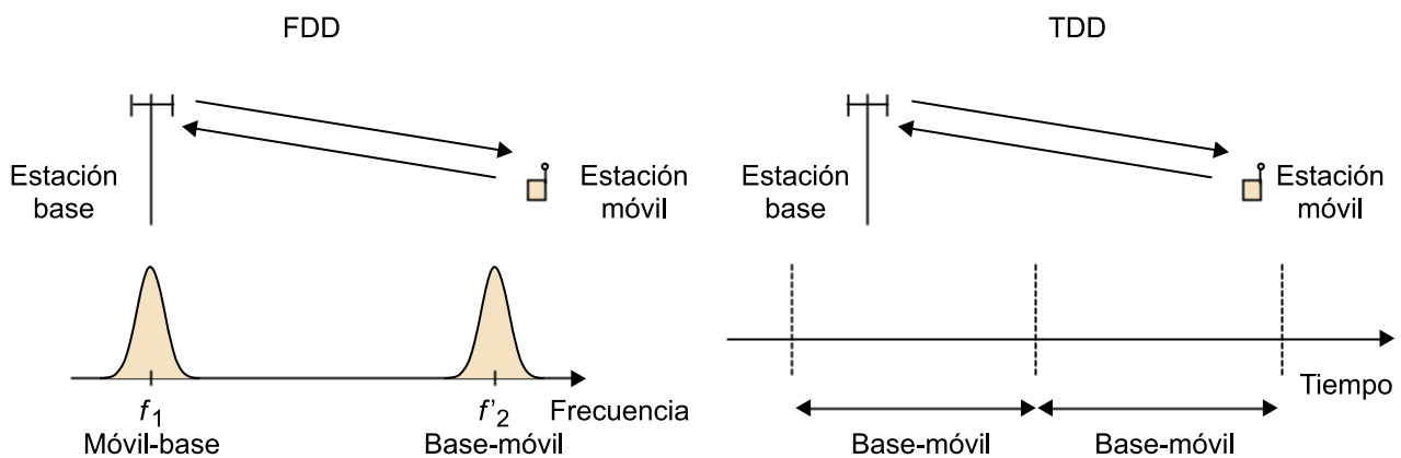
Figura 18. Esquemas de dúplex básicos
