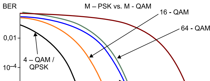
Figura 43. Probabilidad de error de bit (BER) en escala logarítmica de las modulaciones QPSK, 4-QAM, 16-QAM, 16-PSK, 64-QAM, 16-PSK y 64-PSK
