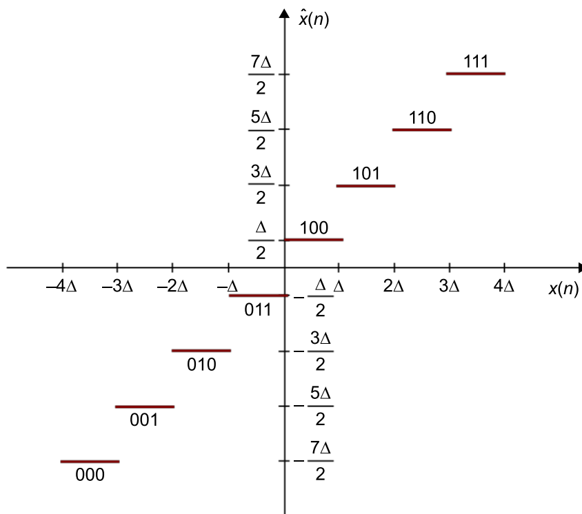
Figura 3. Representación de un posible esquema de cuantificación de ocho niveles (3 bits)
