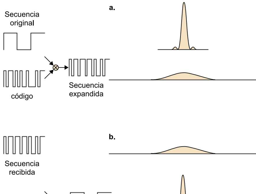
Figura 17. Acceso múltiple por división de código (CDMA)
