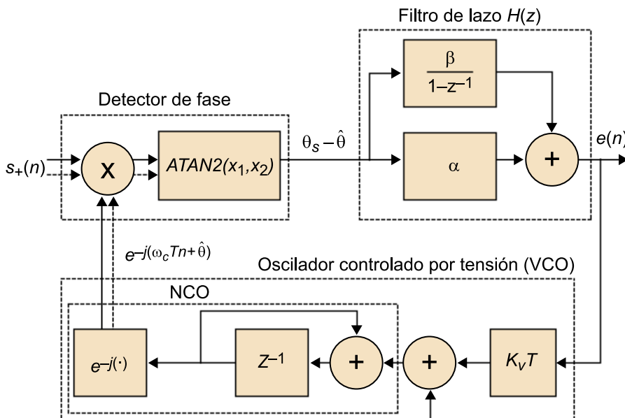
Figura 23. Estructura de un PLL digital
