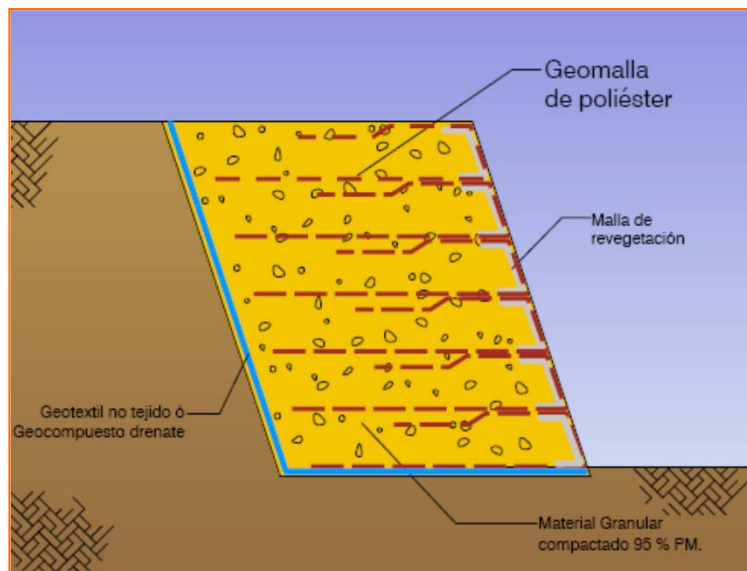
Estructura de muro con geomalla
