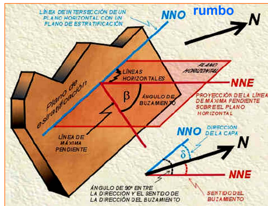
Caracterización de buzamiento
