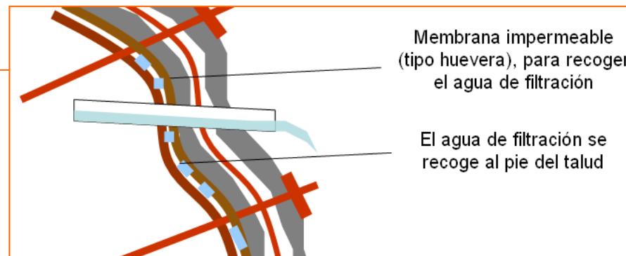
Variante con membrana impermeable
