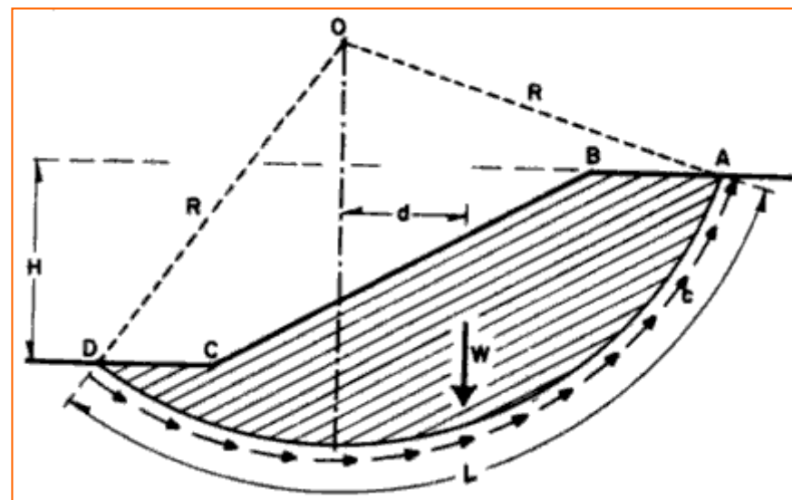
Esquema de rotura circular para talud en suelo con cohesión únicamente
