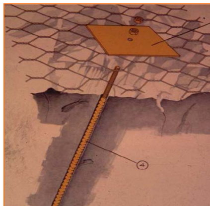
Uso de mallas para detención de bloques / Esquema anclaje de malla
