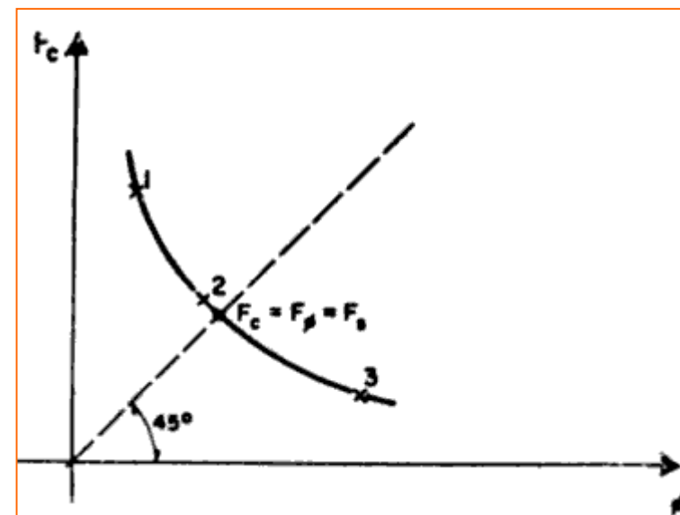
Método gráfico de Taylor para obtener F_\phi = F_c = FS
