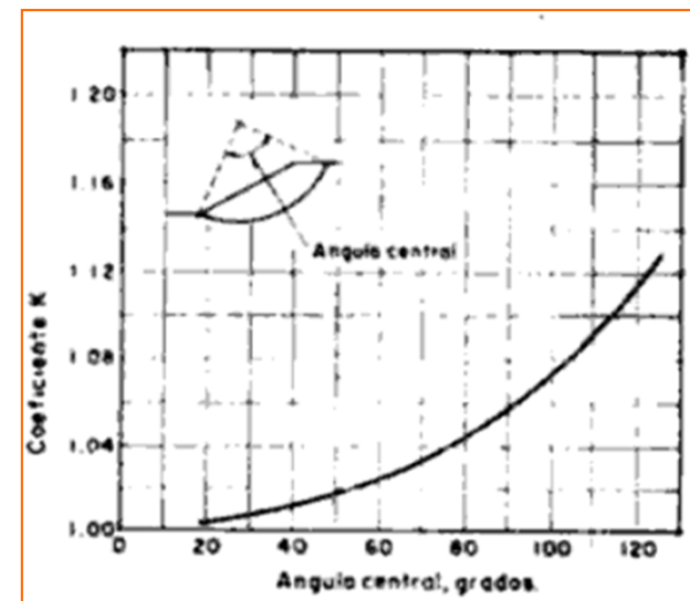
Gráfico de Taylor para obtener K
