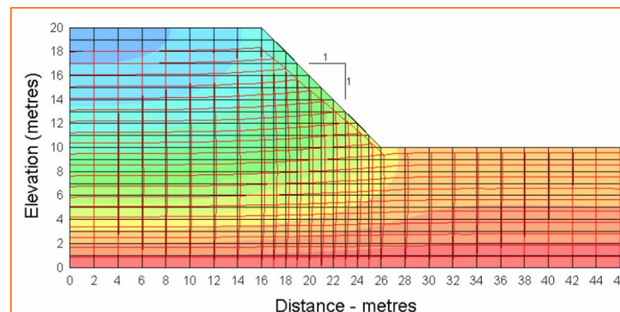
Malla típica de elementos finitos
