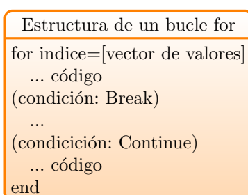
Figura 2.13: Esquema general de la estructura de un bucle for los términos escritos entre paréntesis son opcionales.
