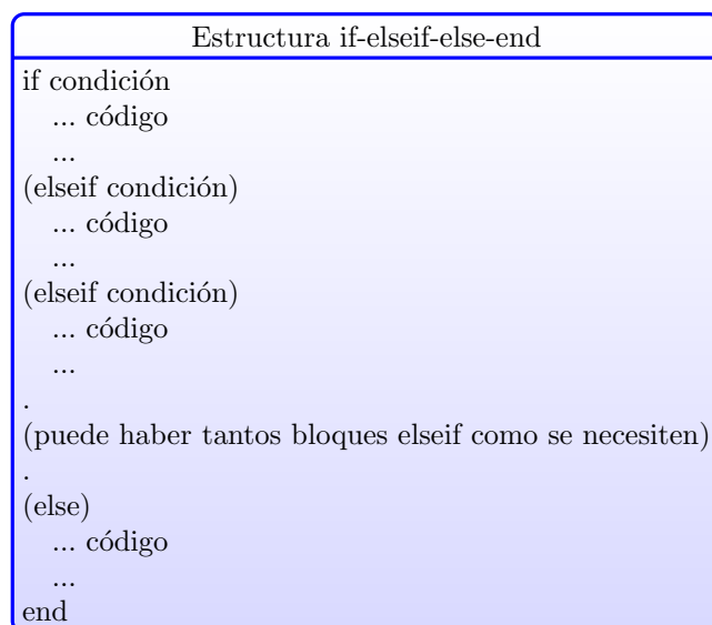
Figura 2.11: Esquema general de la estructura de flujo condicional if los términos escritos entre paréntesis son opcionales.
