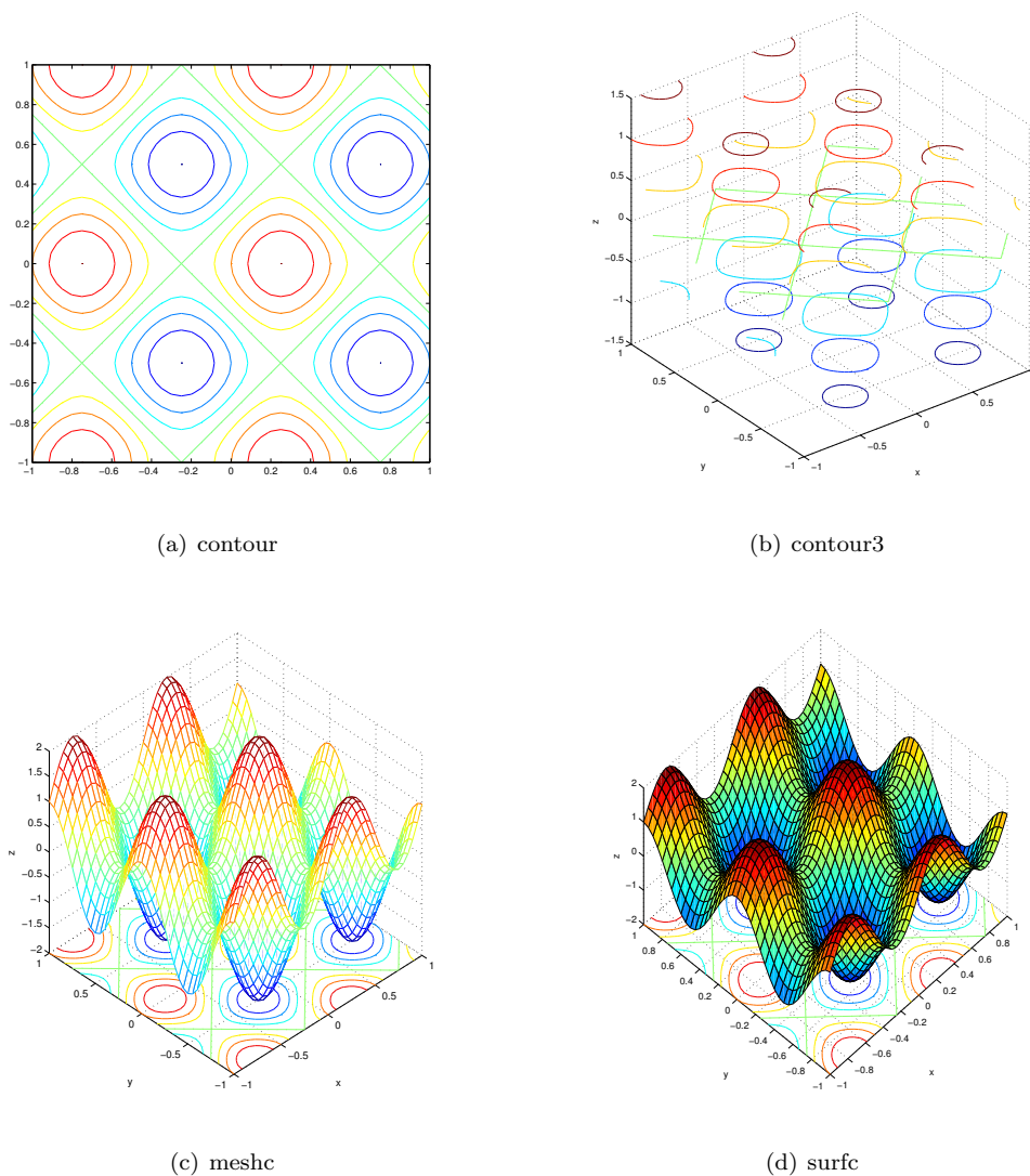
Figura 2.38: Comparación entre los resultados de contour , contour3 , meshc y surf , para la obtención de las curvas de nivel de una superficie.
