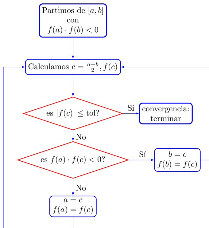
Figura 4.3: Diagrama de flujo del método de la bisección
