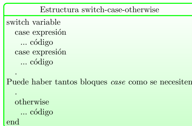
Figura 2.12: Esquema general de la estructura switch-case-otherwise
