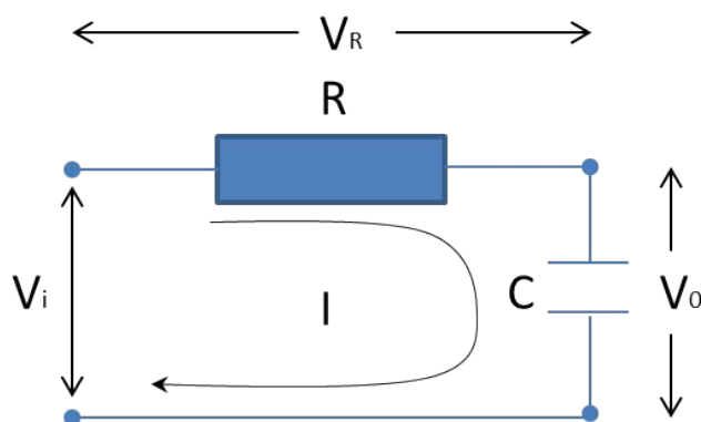
Figura 8.7: Circuito RC
