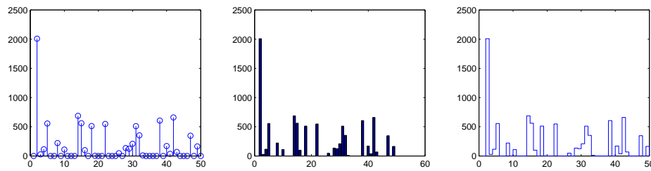
Figura 2.26: Comparción entre los comandos stem , bar y stairs representando la misma colección de datos.
