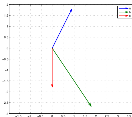
Figura 5.1: Representación gráfica de vectores en el plano
