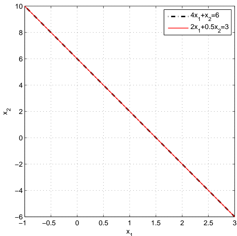
Figura 6.3: Sistema de ecuaciones con infinitas soluciones
