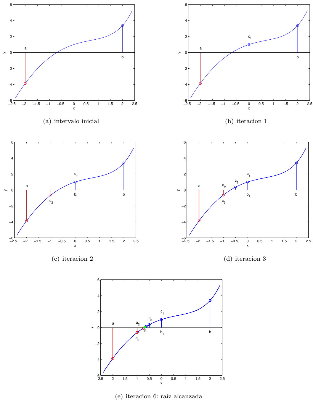
Figura 4.4: proceso de obtención de la raíz de una función por el método de la bisección
