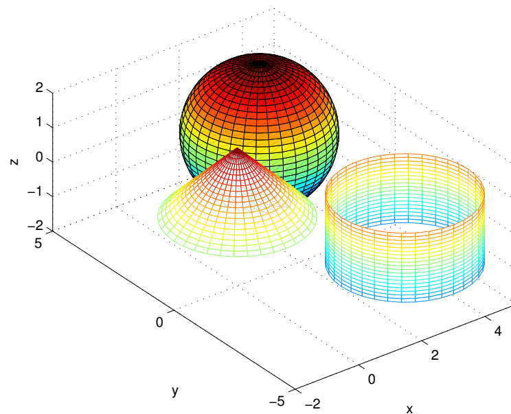
Figura 2.37: retícula con simetría circular
