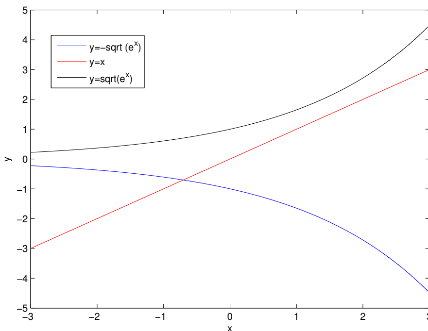
Figura 4.16: g(x) = \pm\sqrt{e^x} , Solo la rama negativa tiene un punto fijo.
