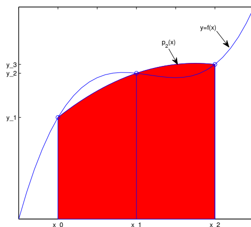
Figura 8.5: Interpretación gráfica de la fórmula 1/3 de Simpson.
