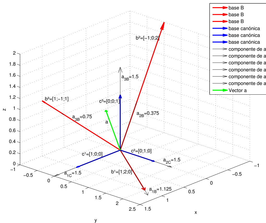
Figura 5.7: Representación gráfica del vector a , en las base canónica \mathcal{C} y en la base \mathcal{B}
