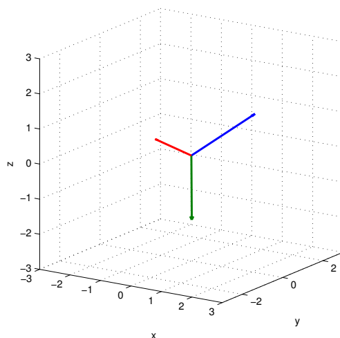
Figura 5.2: Representación gráfica de vectores en el espacio
