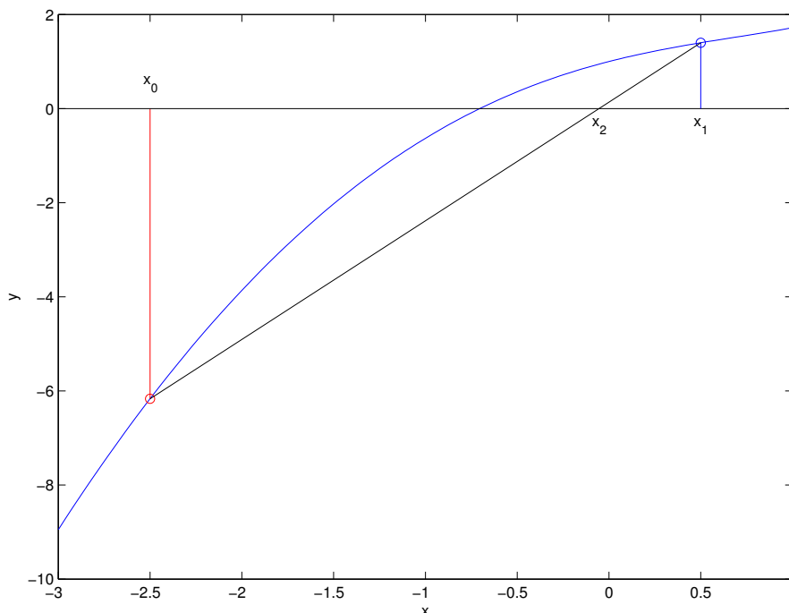
Figura 4.11: Recta secante a la función f(x) en los puntos x_0 y x_1
