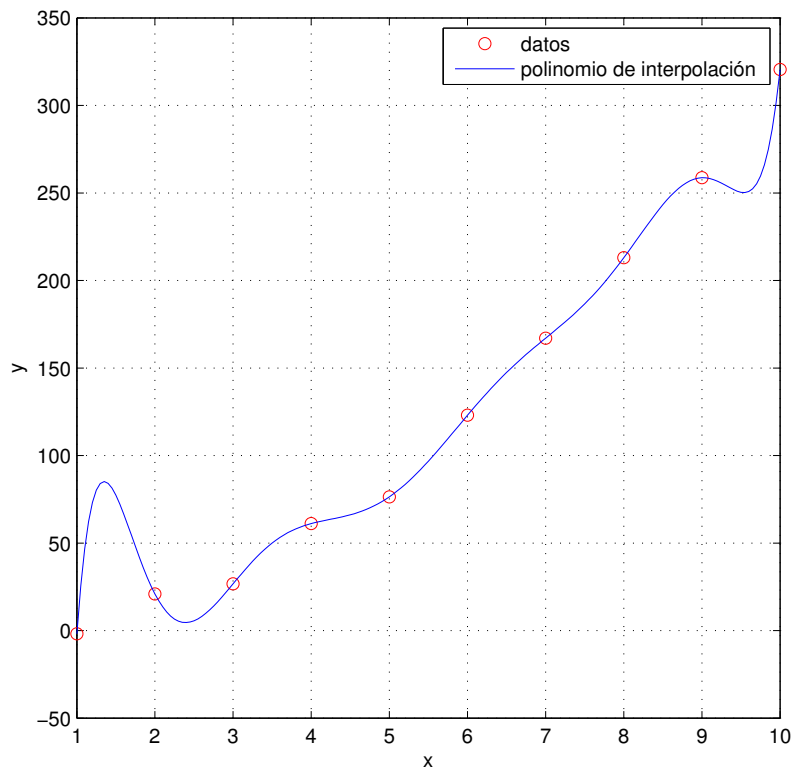
Figura 7.3: Polinomio de interpolación de grado nueve obtenido a partir de un conjunto de diez datos
