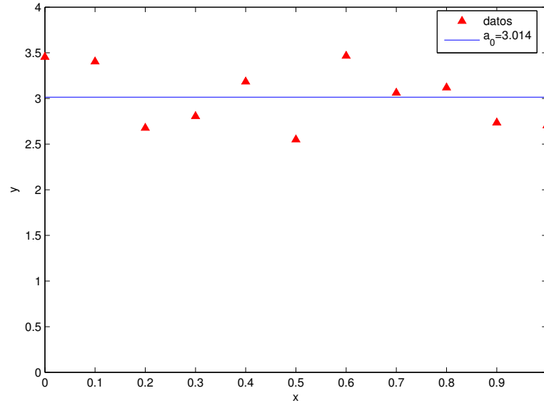
Figura 7.6: Polinomio de mínimos cuadrados de grado 0
