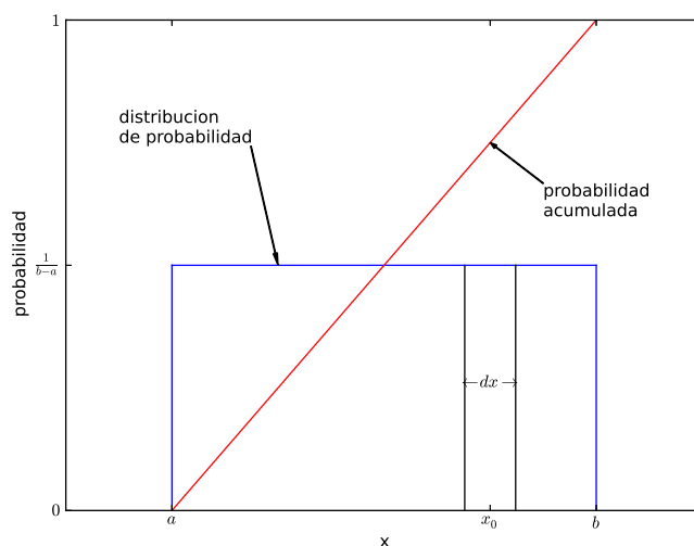
Figura 9.5: Distribución de probabilidad uniforme para un intervalo [a, b] y probabilidad acumulada correspondiente
