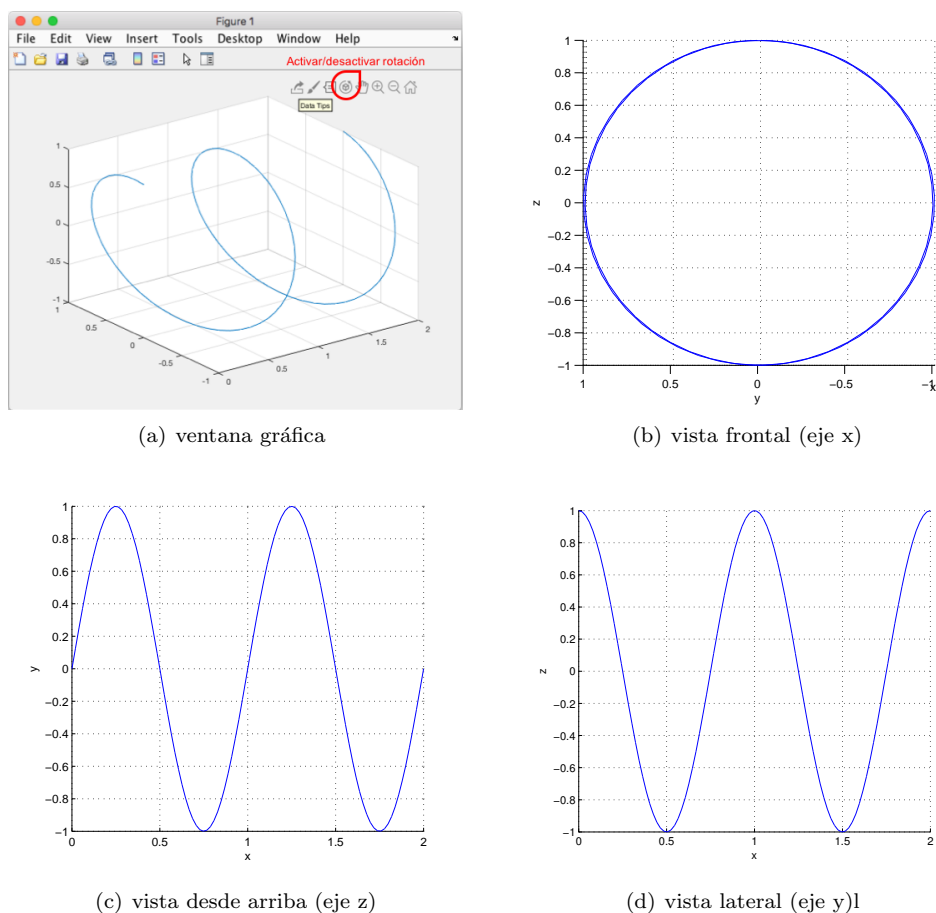
Figura 2.31: Gráfico en 3D y rotaciones.
