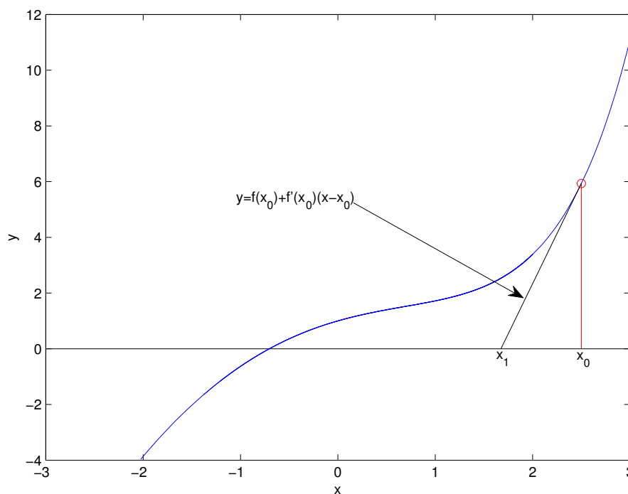
Figura 4.8: Recta tangente a la función f(x) en el punto x_0
