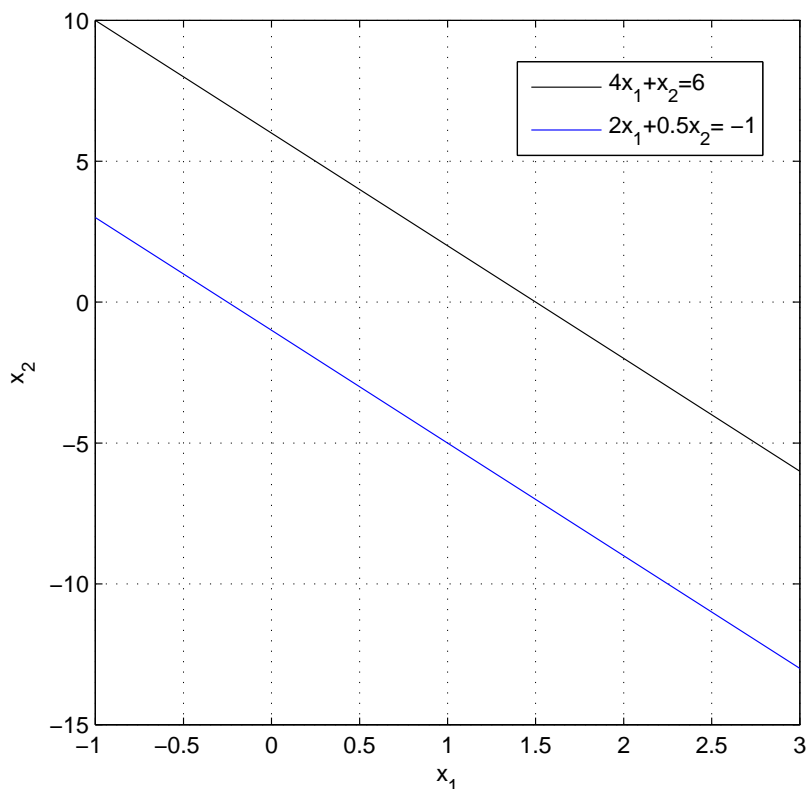
Figura 6.2: Sistema de ecuaciones sin solución
