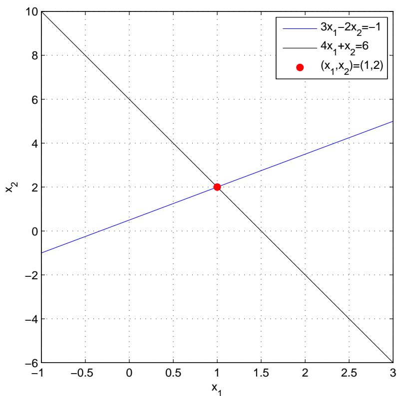
Figura 6.1: Sistema de ecuaciones con solución única
