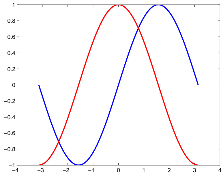
Figura 2.20: gráficas de las funciones seno y coseno en el intervalo (-\pi, \pi) . Representadas en la misma figura, usando el comando hold on .
