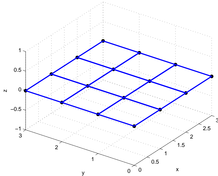
Figura 2.32: Retícula para representar superficies. Los puntos negros son los nodos definidos por las matrices X_m e Y_m .
