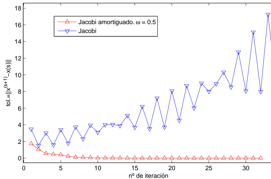
Figura 6.6: Evolución de la tolerancia para un mismo sistema empleando el método de Jacobi (diverge) y el de Jacobi amortiguado (converge).
