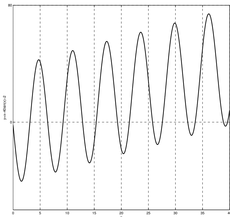
Figura 4.1: Ejemplo de ecuación de Kepler para a = 40 y b = 2
