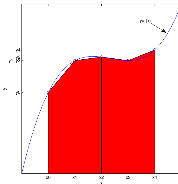
Figura 8.4: Interpretación gráfica de la fórmula extendida del trapecio.
