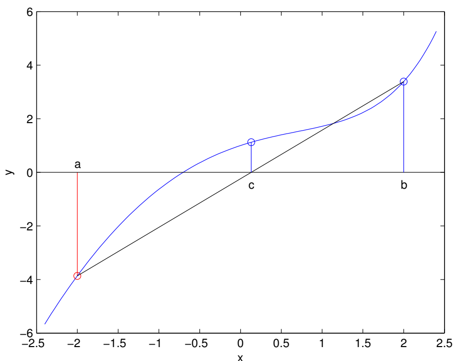
Figura 4.5: Obtención de la recta que une los extremos de un intervalo [a, b] que contiene una raíz de la función
