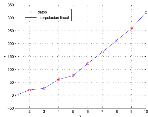
(b) Interpolación lineal
