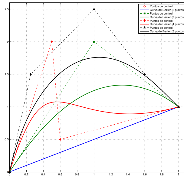
Figura 7.9: Curvas de Bézier trazadas entre los puntos P_0 = (0, 0) y P_n = (2, 1) , variando el número y posición de los puntos de control.
