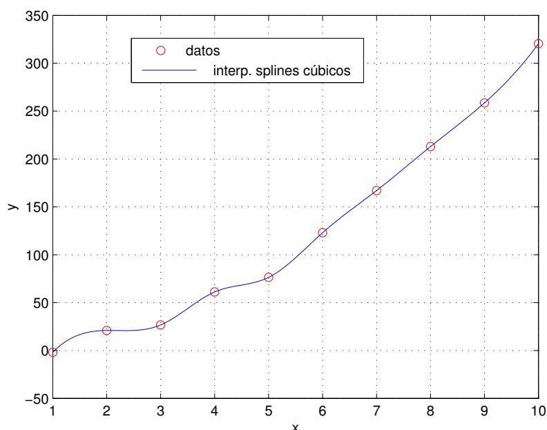
Figura 7.5: Interpolación mediante spline cúbico de los datos de la figura 7.3
