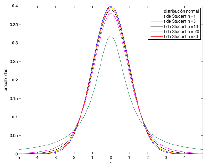
Figura 9.13: Comparación entre las distribuciones t de Student de 1, 5, 10, 20 y 30 grados de libertad y la distribución normal.
