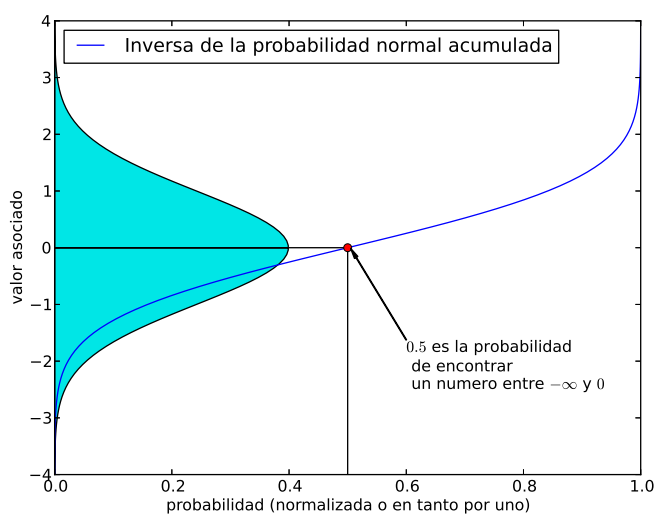
Figura 9.11: Función inversa de probabilidad normal acumulada s
