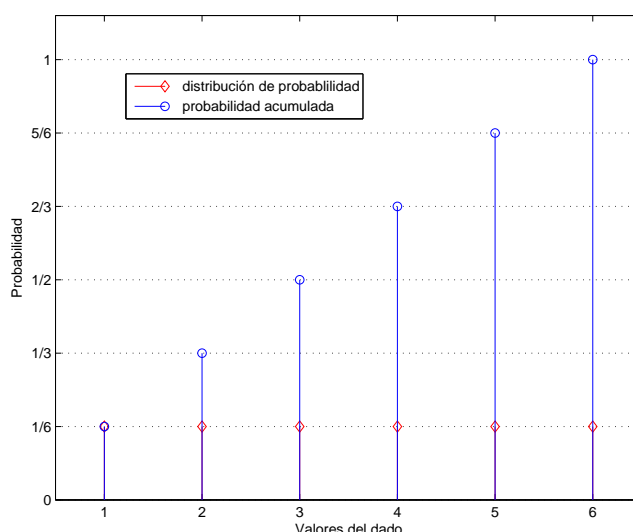
Figura 9.3: Distribución de probabilidad y probabilidad acumulada de los resultados de lanzar un dado al aire.
