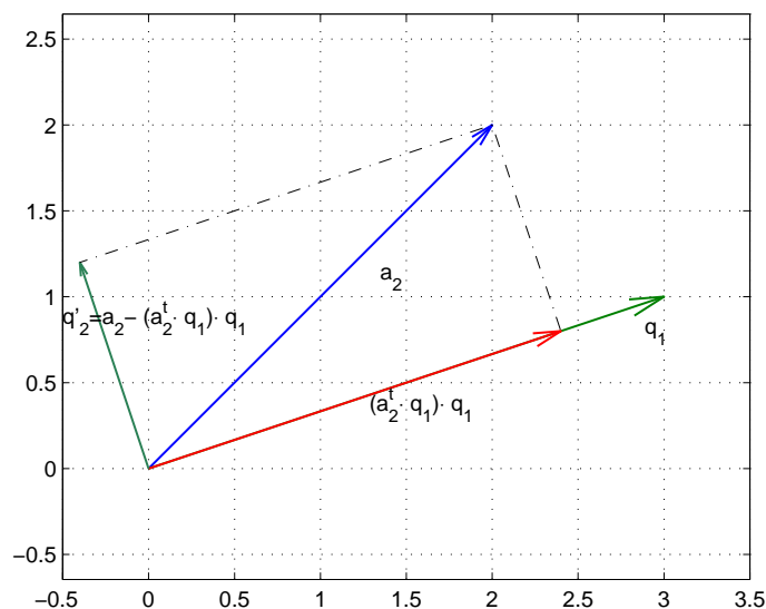
Figura 5.10: Obtención de un vector ortogonal
