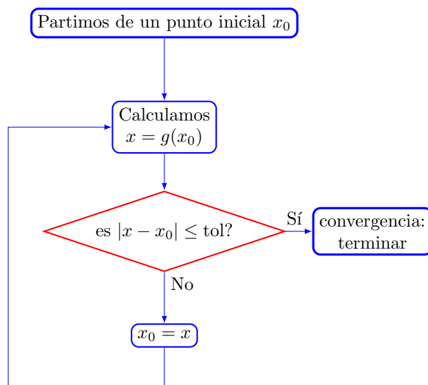
Figura 4.15: Diagrama de flujo del método del punto fijo. Nótese que la raíz obtenida corresponde a la función f(x) = g(x) - x
