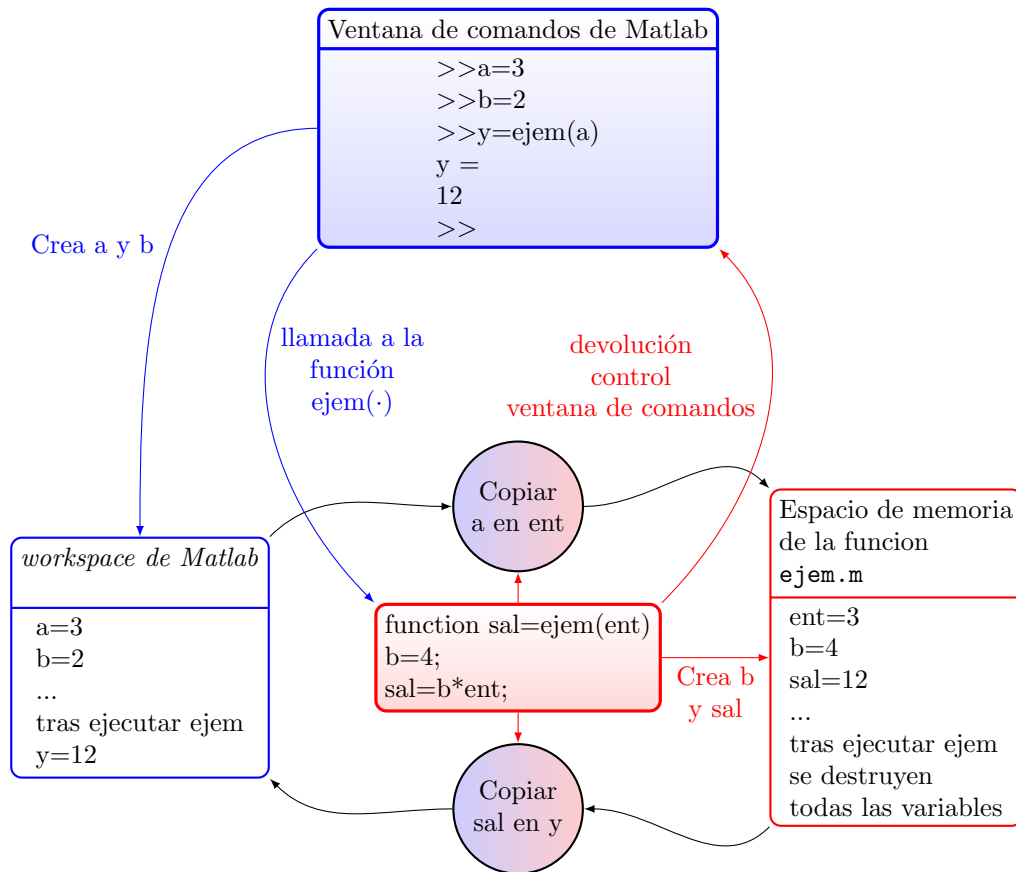
Figura 2.6: Ejemplo de uso de memoria y ámbito de variables durante la ejecución de una función
