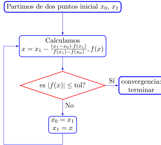
Figura 4.12: Diagrama de flujo del método de la secante
