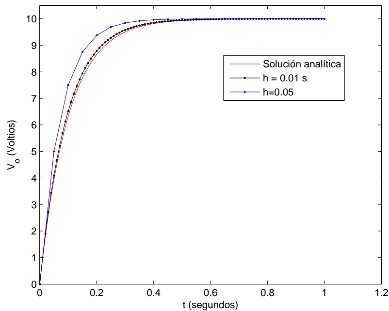
Figura 8.8: Comparación entre los resultados obtenidos mediante el método de Euler para dos pasos de integración h = 0,05 y h = 0,001 y la solución analítica para el voltaje V_o de un condensador durante su carga.
