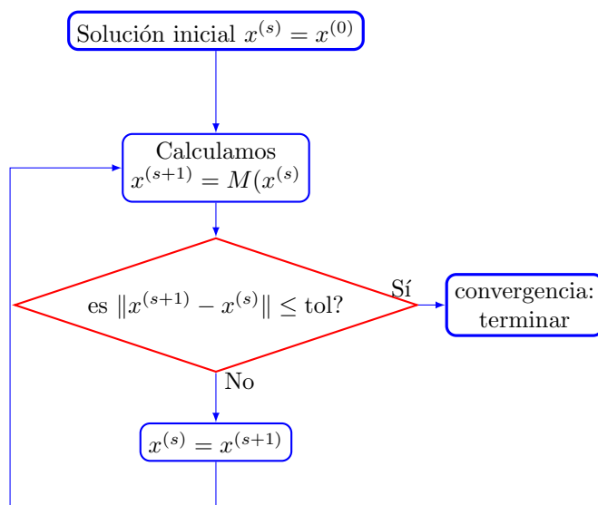
Figura 6.4: Diagrama de flujo general de los métodos iterativos para resolver sistemas de ecuaciones. La función M(x) es la que especifica en cada caso el método.
