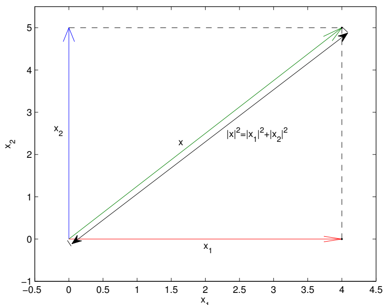
Figura 5.3: interpretación geométrica de la norma de un vector
