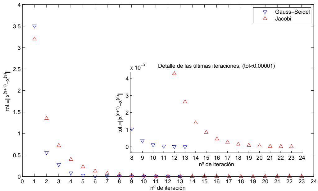
Figura 6.5: evolución de la tolerancia (módulo de la diferencia entre dos soluciones sucesivas) para un mismo sistema resuelto mediante el método de Gauss-Seidel y el método de Jacobi
