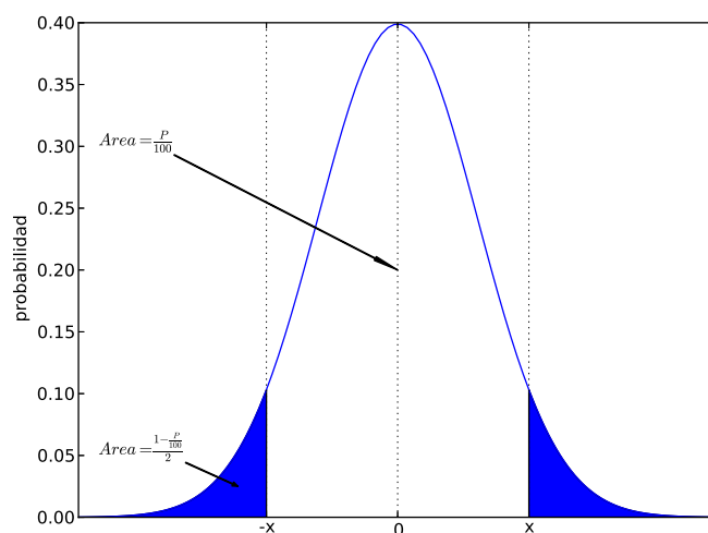
Figura 9.12: Intervalo de probabilidad P %
