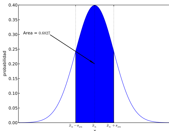
Figura 9.10: Intervalo de confianza del 68,27%
