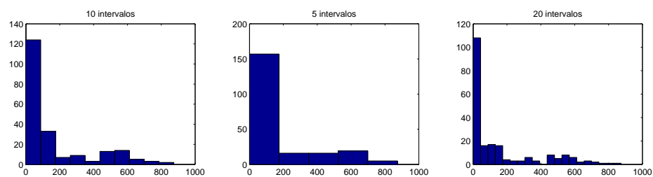
Figura 2.27: histogramas del número de automóviles por cada 1000 habitantes para 213 países
