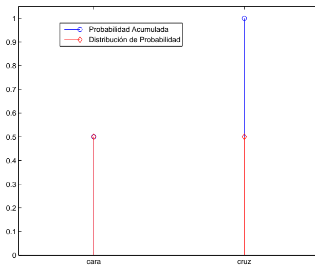
Figura 9.2: Distribución de probabilidad y probabilidad acumulada de los resultados de lanzar una moneda al aire.
