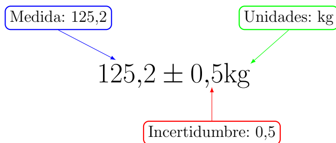
Figura 9.9: Modo correcto de expresar una medida experimental
