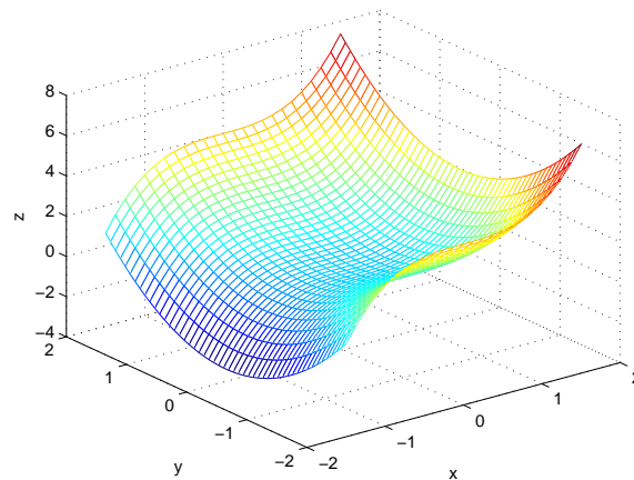
(a) Función z = x^3 + y^2 representada con mesh
