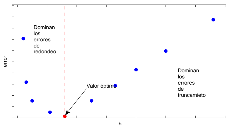
Figura 8.1: Variación del error cometido al aproximar la derivada de una función empleando una fórmula de diferenciación de dos puntos.
