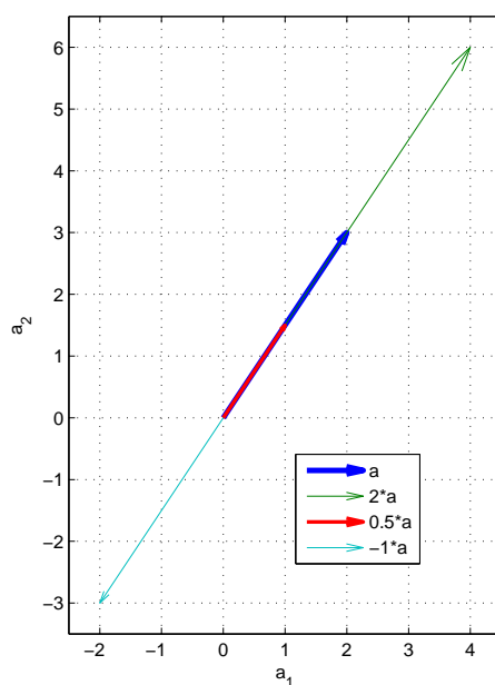
Figura 5.4: efecto del producto de un escalar por un vector
