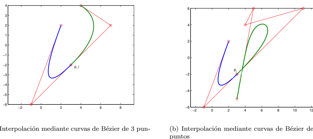
Figura 7.12: Interpolación de tres puntos mediante dos curvas de Bézier
