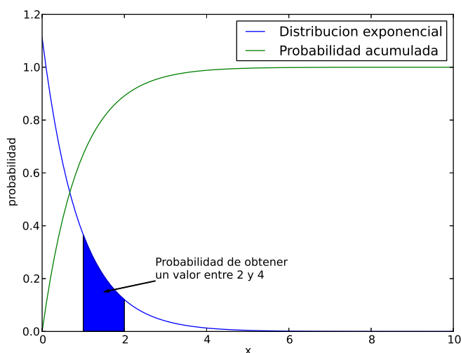
Figura 9.6: Distribución de probabilidad exponencial
