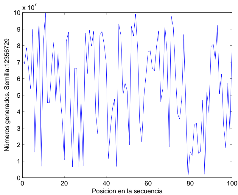
Figura 9.1: Secuencia de 100 números pseudoaleatorios generada mediante el método middle square . 0.4
