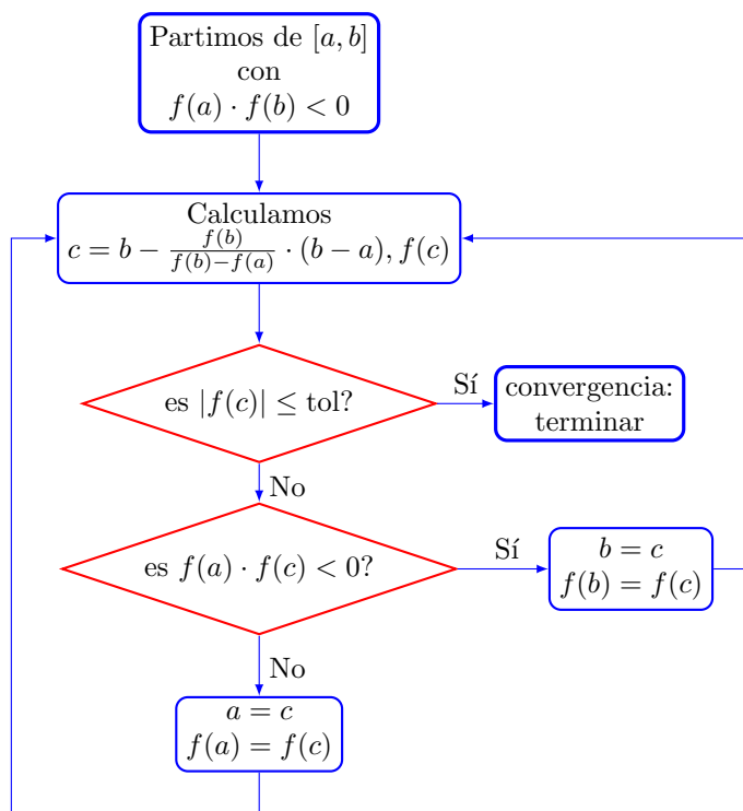
Figura 4.6: Diagrama de flujo del método de interpolación lineal
