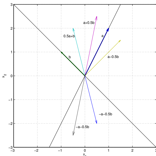
Figura 5.5: Representación gráfica de los vectores a = (1, 2) , b = (-1, 1) y algunos vectores, combinación lineal de a y b .
