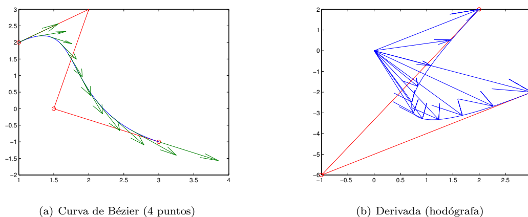
Figura 7.11: Curva de Bézier y su derivada con respecto al parámetro del polinomio de Bernstein que la define: t \in [0, 1]
