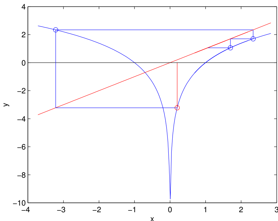
Figura 4.18: primeras iteraciones de la obtención de la raíz de la función f(x) = e^x - x^2 aplicando el método del punto fijo sobre la función g(x) = \ln(x^2) .
