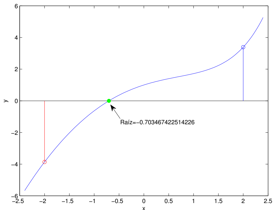
Figura 4.2: Ilustración del teorema de Bolzano
