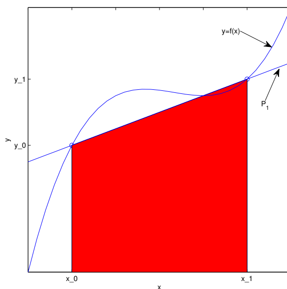
Figura 8.3: Interpretación gráfica de la fórmula del trapecio.
