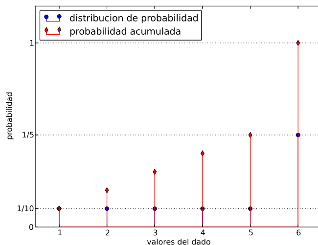
Figura 9.4: Distribución de probabilidad y probabilidad acumulada de los resultados de lanzar un dado trucado al aire.
