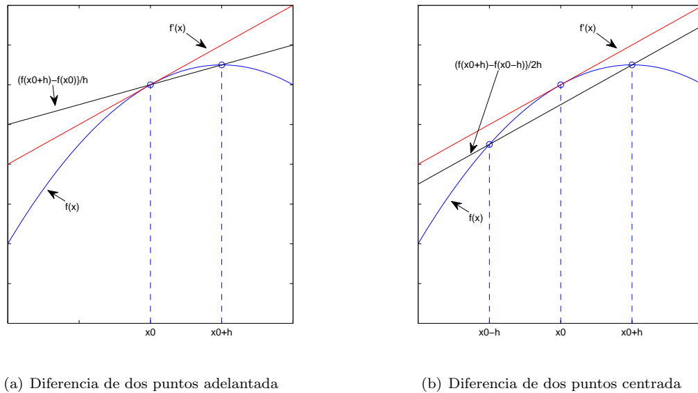
Figura 8.2: Comparación entre las aproximaciones a la derivada de una función obtenidas mediante las diferencias de dos puntos adelantada y centrada
