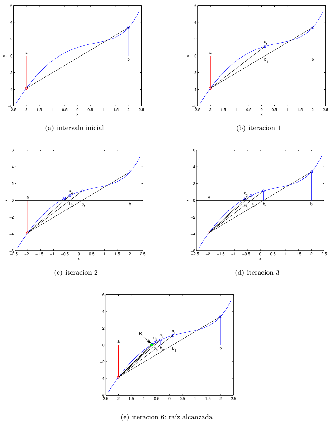
Figura 4.7: Proceso de obtención de la raíz de una función por el método de interpolación lineal
