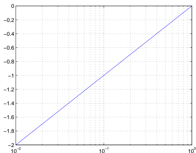
Figura 2.23: Representación de la función y = \log_{10}(x) empleando el comando semilogx
