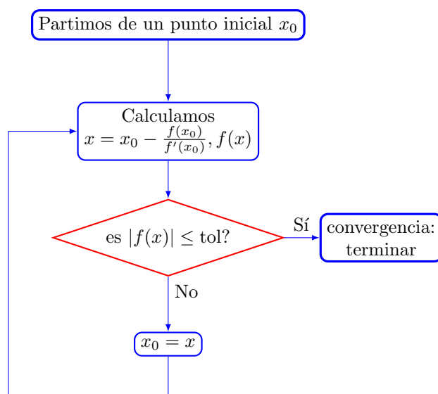
Figura 4.9: Diagrama de flujo del método de Newton-Raphson
