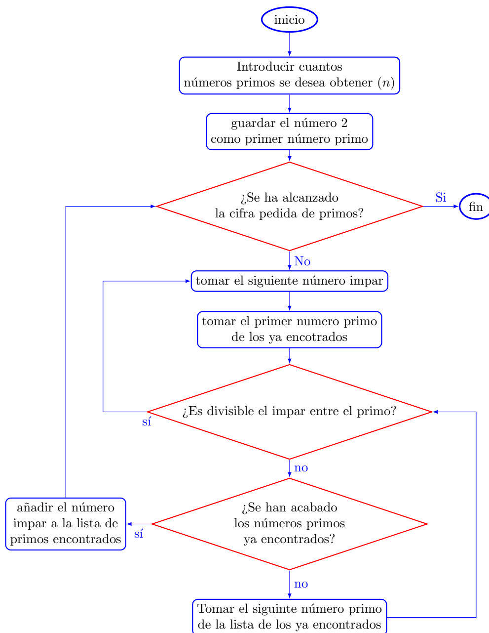
Figura 2.16: Diagrama de flujo para el problema de los números primos
