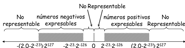
Figura 3.3: Números representables y desbordamientos en el estándar IEEE 754 de precisión simple.
