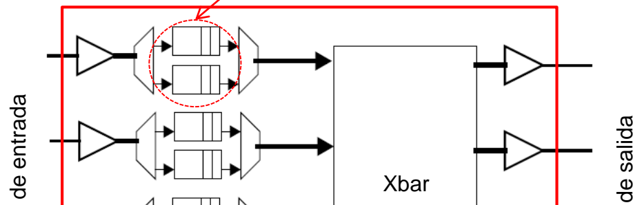
Conmutador con 2 canales virtuales por puerto de entrada
