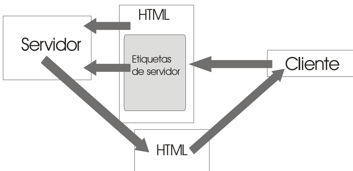
Ilustración 36, Esquema de las tecnologías de servidor. El servidor traduce las etiquetas y devuelve al cliente el código HTML resultado de esas etiquetas
