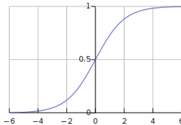
Figura 23: Función logística para una variable regresora 35
