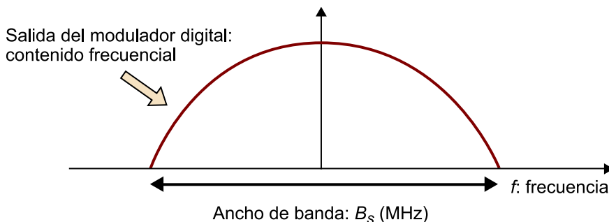
Figura 5. Ocupación espectral en banda base de una modulación digital
