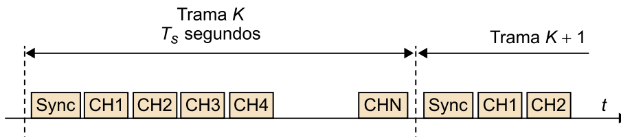
Figura 2. Esquema de multiplexado/acceso múltiple TDM/A
