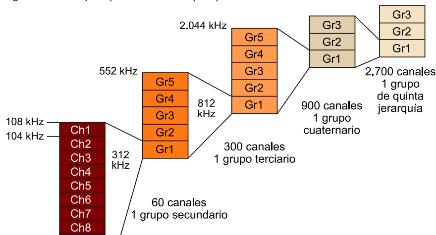
Figura 5. Niveles jerárquicos de un múltiplex por división en frecuencia
