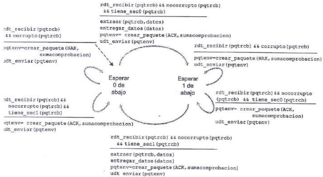
Figura 3.12 • Lado receptor de rdt2.1.
