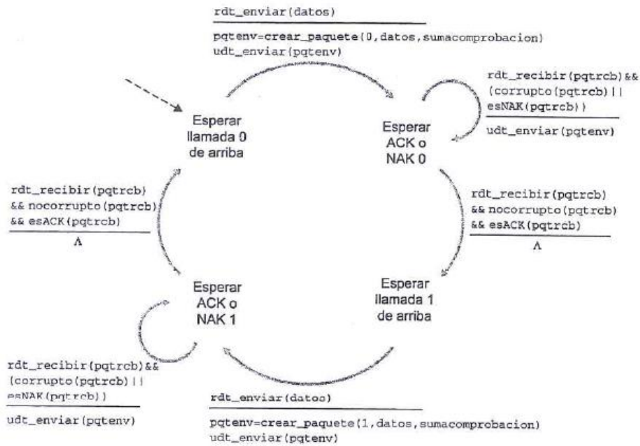
Figura 3.11 • Lado emisor de rdt2.1.
