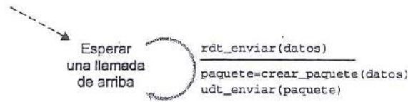
a. rdt1.0: lado emisor
