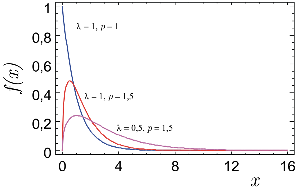
Figura 2: Distribución Gamma para diferentes valores de \lambda y p .
