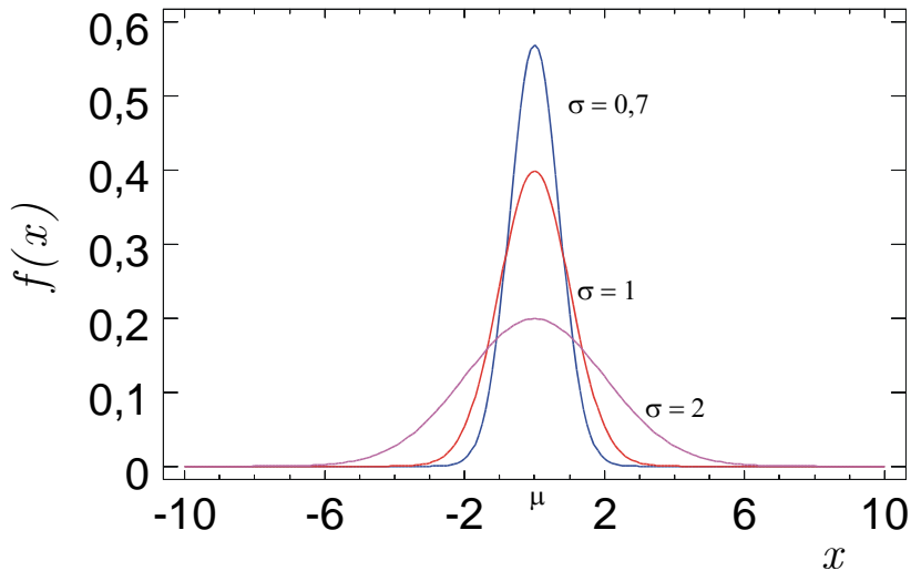
Figura 1: Distribución Normal para diferentes valores de \sigma
