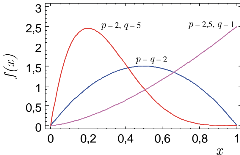
Figura 3: Distribución Beta para diferentes valores de p y q
