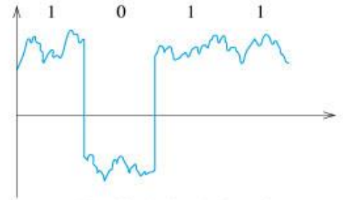
(d) Digital signal plus noise
