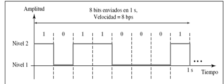
a. Una señal digital con dos niveles
