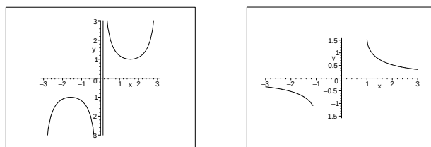
Figura A.8: Gráficas de \csc(x) y \operatorname{arccsc}(x)
