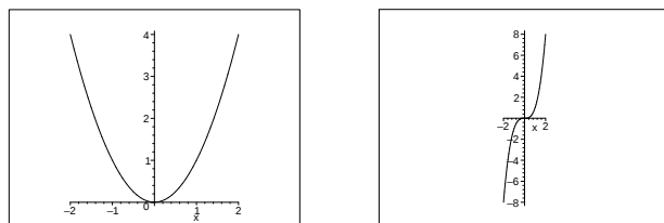
Figura A.1: Gráficas de x^2 y x^3
