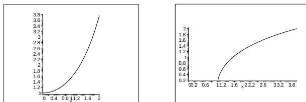
Figura A.12: Gráficas de \operatorname{cosh}(x) y \operatorname{argcosh}(x)
