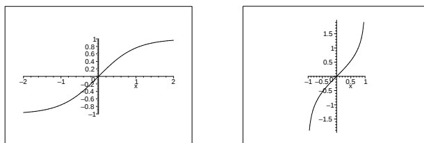
Figura A.13: Gráficas de \operatorname{tanh}(x) y \operatorname{argtanh}(x)
