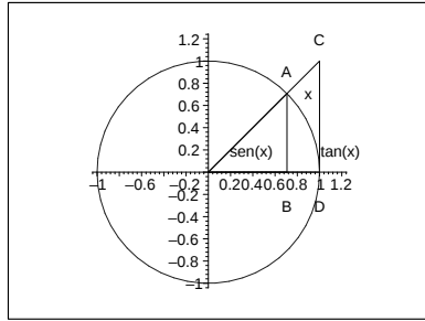
Figura 6.5: El ángulo x , \text{sen}(x) y \tan(x) .
