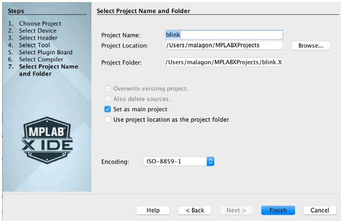
Figura 11. Nombre de proyecto y establecer como Main Project
