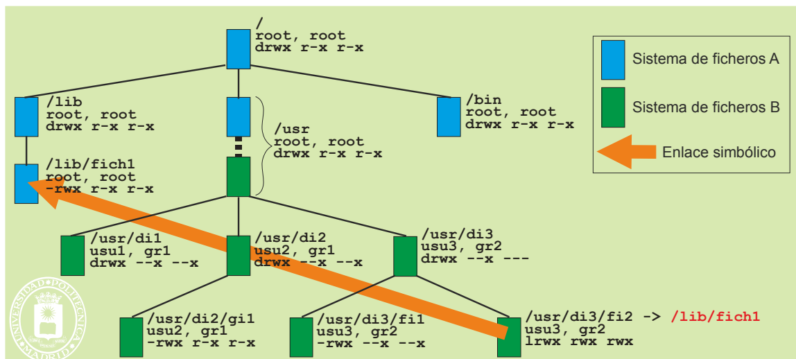
Figura 5.37 Ejemplo de análisis de permisos. Para abrir /usr/di3/fi2 se comprueban los permisos de: / (raíz SF A), /usr/ (raíz SF B), /di3/ , / (raíz SF A), /lib/ , /fich1 . No se comprueban los permisos almacenados en el nodo- i de /fi2 ni los del nodo- i original de /usr/ .
