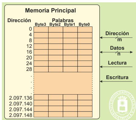
Figura 1.3 La Unidad de memoria está compuesta por un conjunto de celdas iguales que se seleccionan mediante una dirección. Las señales de control de lectura y escritura determinan la operación a realizar.
