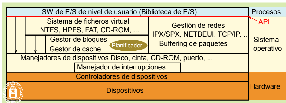
Figura 5.1 Principales capas de un sistema de E/S.
