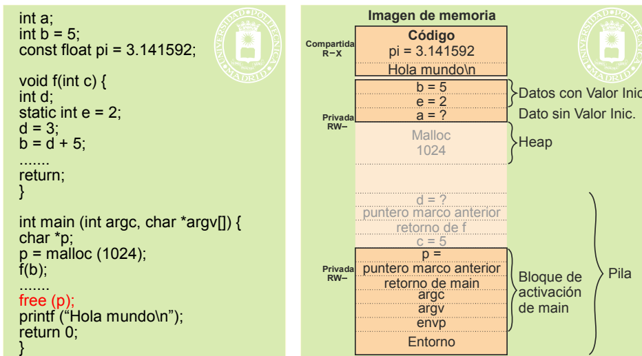
Figura 4.43 Imagen de memoria del proceso al ejecutarse el free .
