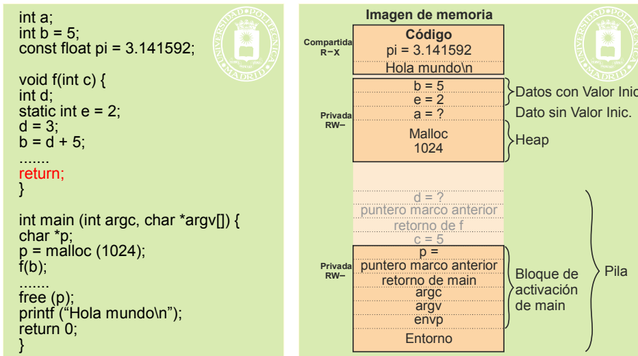
Figura 4.42 Imagen de memoria del proceso al ejecutarse el return de la función f .
