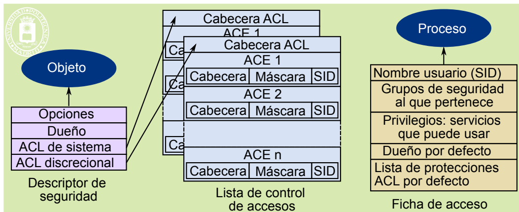
Figura 5.35 En Windows la seguridad está basada en las fichas de acceso asociada a cada usuario, más los descriptores de seguridad asociado a cada objeto. El descriptor de seguridad apunta a dos listas de control de accesos: una de sistema y otra discrecional.
