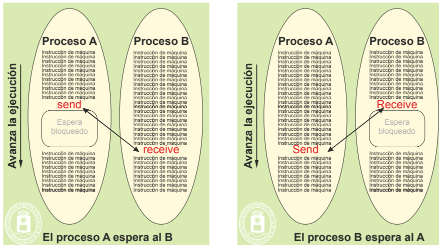
Figura 2.17 Comunicación sincrónica entre procesos.
