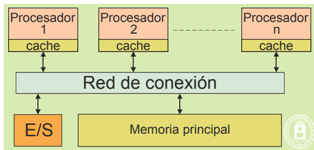
Figura 1.21 Estructura de un multiprocesador.
