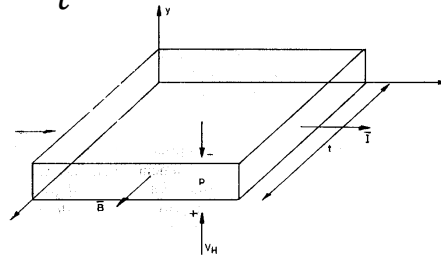
Con semiconductor tipo P.
