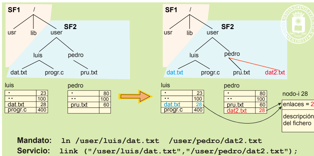
Figura 5.17 Implementación de enlaces físicos en UNIX. Se crea un nuevo fichero dat2.txt en el directorio pedro.
