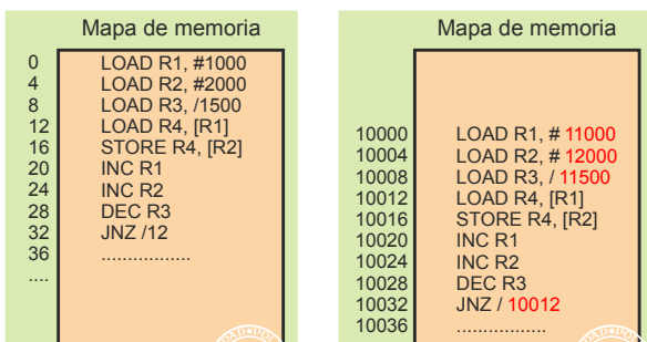
Figura 4.30 Reubicación de un programa preparado para la posición 0 si se carga en la posición 10.000.
