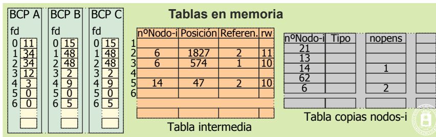
Figura 5.32 Cambios en las tablas de descriptores de ficheros, intermedia y nodos-i al ejecutar varios servicios de cierre de descriptor de ficheros.
