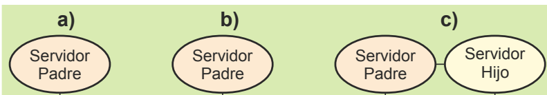
Figura 3.19 Funcionamiento de un proceso servidor.
