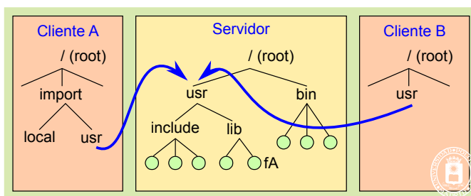
Figura 5.63 Montado de un directorio remoto en dos clientes.
