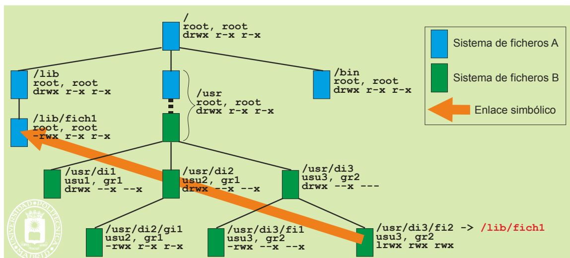
Figura 5.37 Ejemplo de análisis de permisos. Para abrir /usr/di3/fi2 se comprueban los permisos de: "/ (raíz SF A), "/usr/" (raíz SF B), "di3/" , "/ (raíz SF A), "lib/" , "fich1" . No se comprueban los permisos almacenados en el nodo- i de "fi2" ni los del nodo- i original de "/usr/" .
