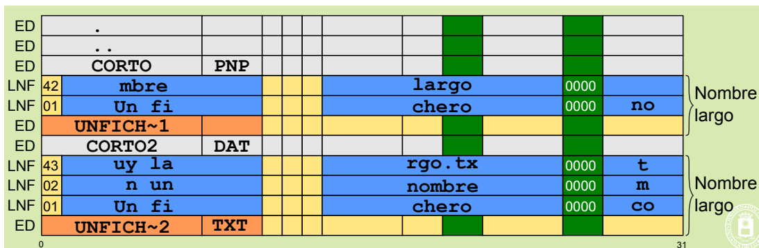
Figura 5.51 Ejemplo de directorio VFAT con 6 entradas, 4 cortas «.», «..», 'CORTO.PNP' y 'CORTO2.DAT', y dos largas.
