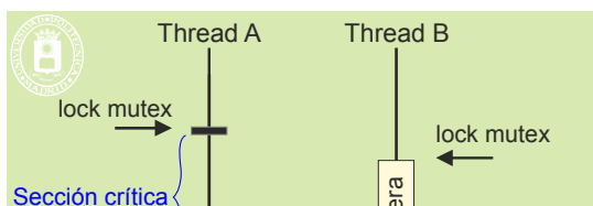
Figura 6.21 Ejemplo de mutex en una sección crítica.
