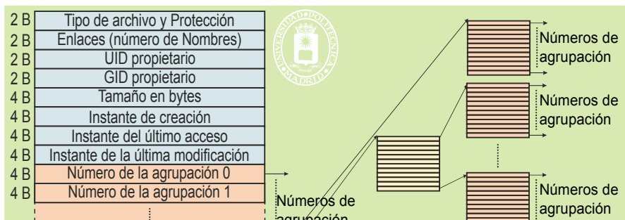
Figura 5.20 Formato del nodo-i clásico de UNIX, concretamente del sistema de ficheros ext2, y las agrupaciones adicionales de indirectos.
