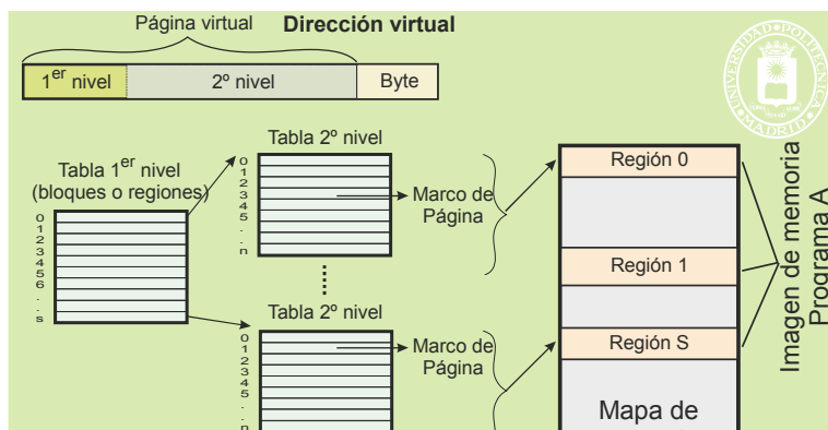
Figura 4.10 Tabla de páginas de dos niveles.
