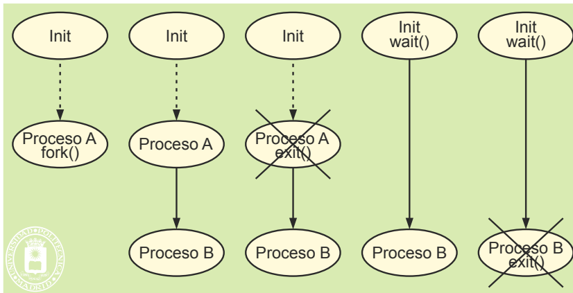
Figura 3.51 En UNIX el proceso init hereda los procesos hijos que se quedan sin padre.
