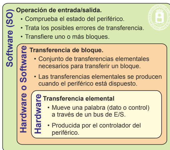
Figura 1.14 Una operación de E/S se suele descomponer en una serie de transferencias de bloques (e.g. sectores del disco). A su vez cada bloque requiere una transferencia elemental por cada palabra de información transferida.
