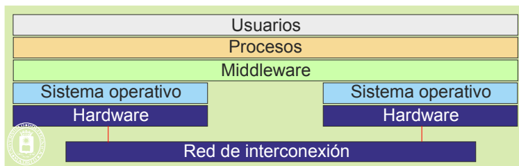
Figura 2.28 Estructura de un middleware.
