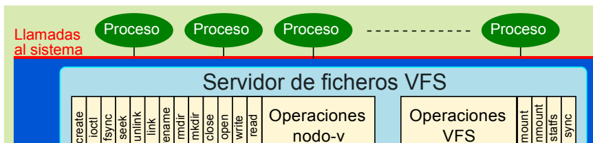
Figura 5.42 El servidor de ficheros virtual ofrece al usuario una visión uniforme de todos los sistemas de ficheros instalados en el computador.
