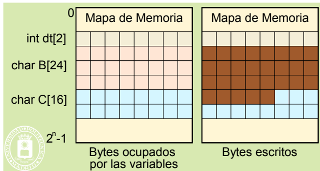
Figura 5.31 Ejemplo de desbordamiento de buffer en una máquina de 64 bits, al ejecutar: read(fd1, B, 30) ; Se escriben los 30 bytes marcados en marrón en la figura. Pero, al tener B un tamaño de 24 bytes se sobrescriben también los 5 primeros bytes de C.
