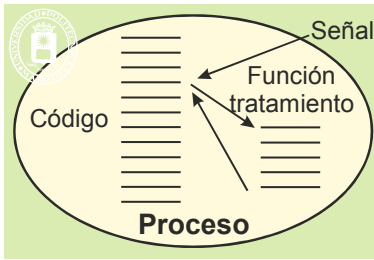
Figura 3.16 Recepción de una señal por parte de un proceso.
