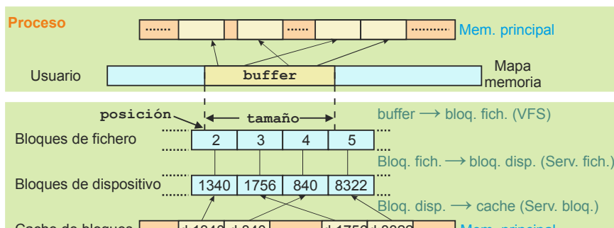
Figura 5.40 Flujo de datos para el caso en el que el servidor de bloques realiza la proyección de bloques de dispositivo a cache.
