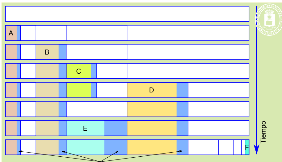
Figura 4.53 Sistema de asignación de memoria buddy binario.
