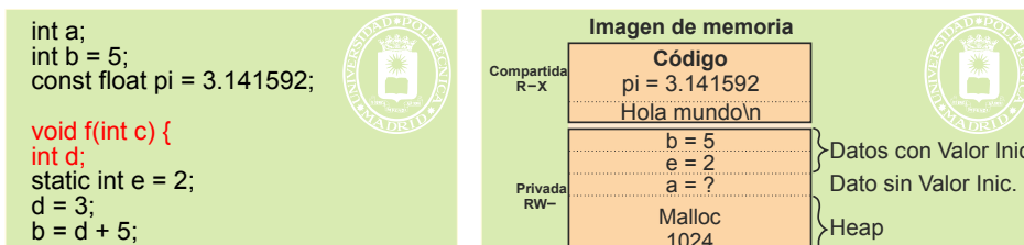
Figura 4.41 Imagen de memoria del proceso al ejecutarse la llamada a la función f.
