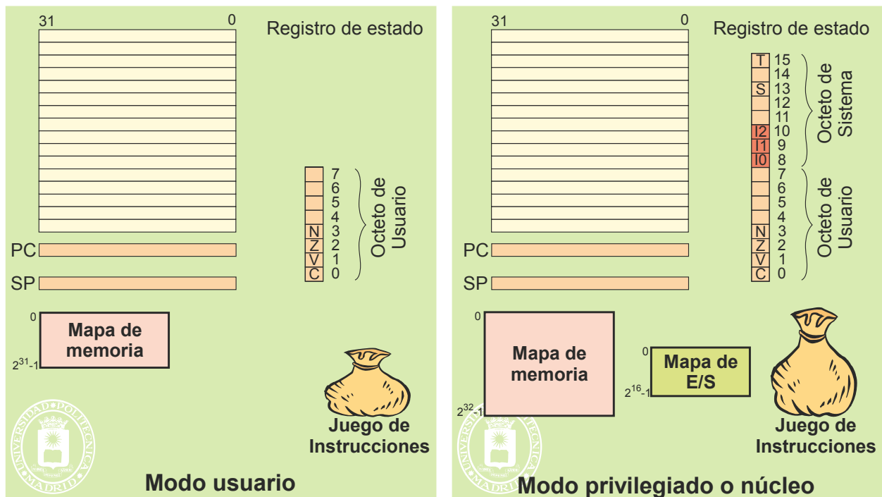
Figura 1.6 Modelos de programación de usuario y de privilegiado.
