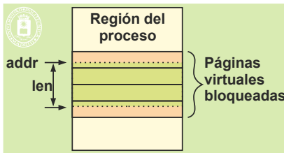
Figura 4.60 El servicio mlock bloquea páginas en memoria principal.
