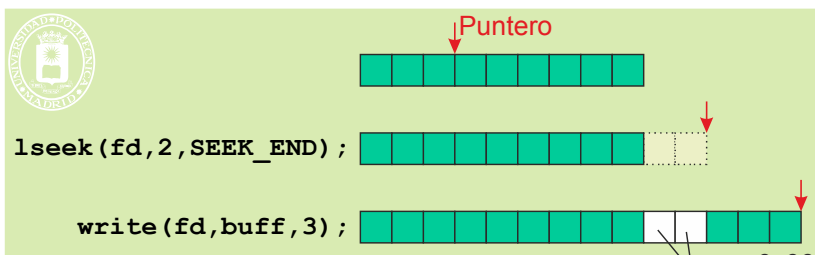
Figura 5.33 Creación de un hueco en un fichero en UNIX.
