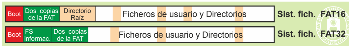
Figura 5.49 Estructura de los sistemas de ficheros FAT16 y FAT32.
