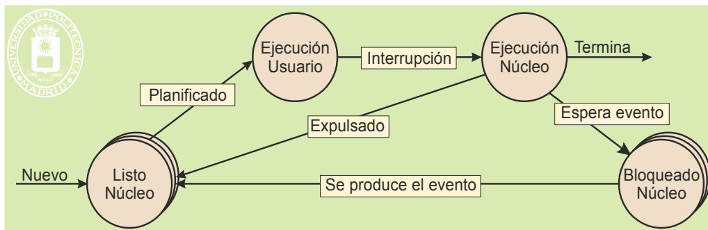
Figura 3.29 Estados básicos del proceso en el caso de ejecución del núcleo dentro del proceso de usuario.
