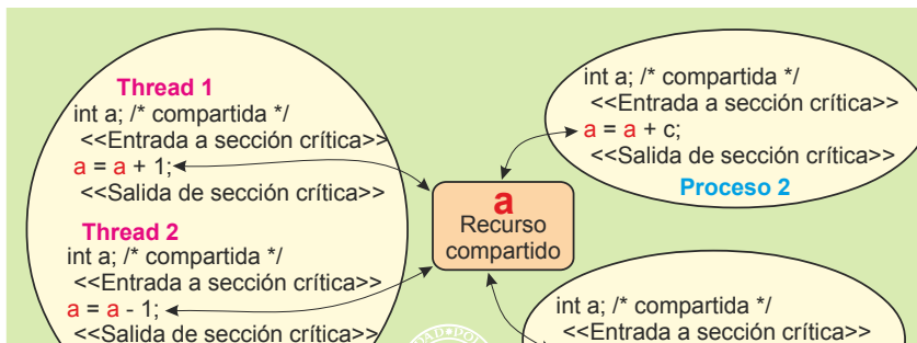
Figura 6.6 Procesos y threads compartiendo una variable a .
