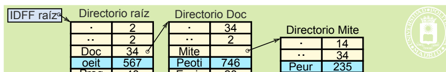
Figura 5.16 El árbol de nombres de un sistema de ficheros se establece como un árbol de tablas directorio.
