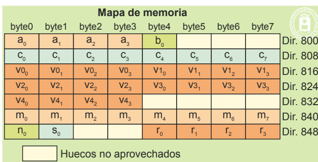
Figura 4.48 La alineación hace que se pierda espacio, por lo que una estructura puede ocupar más espacio de la suma de los espacios necesarios para sus elementos.
