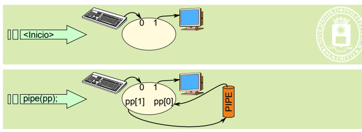
Figura 6.36 Ejecución de mandatos con tuberías en UNIX.
