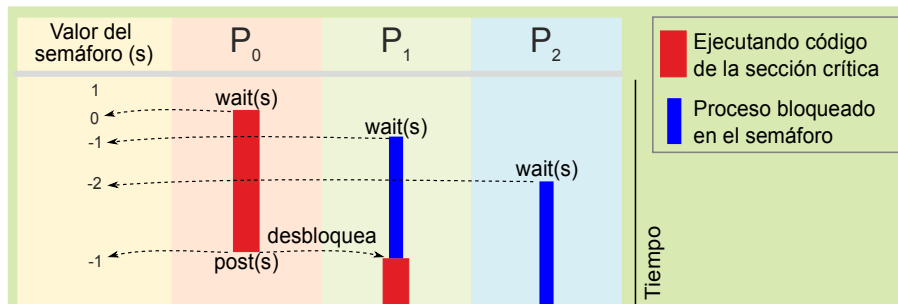
Figura 6.20 Sección crítica con un semáforo binario.
