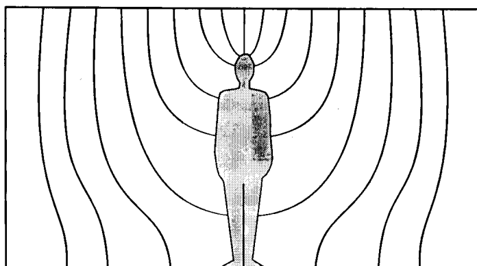
Figura 4.1: Distorsión de las líneas de campo eléctrico terrestre natural causada por la presencia de una persona.
