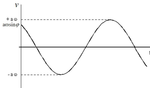
Figura 2.26: Gráfica velocidad-tiempo de un m.a.s.
