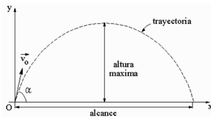
Figura 2.20: Movimiento parabólico.
