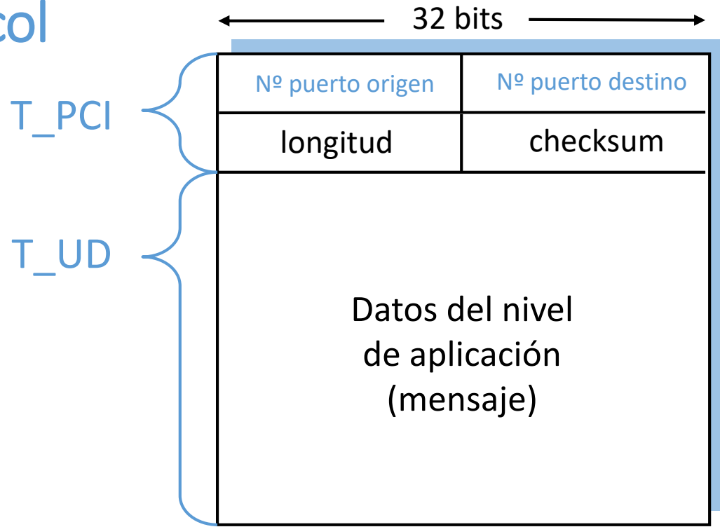
Formato de la T_PDU de UDP
