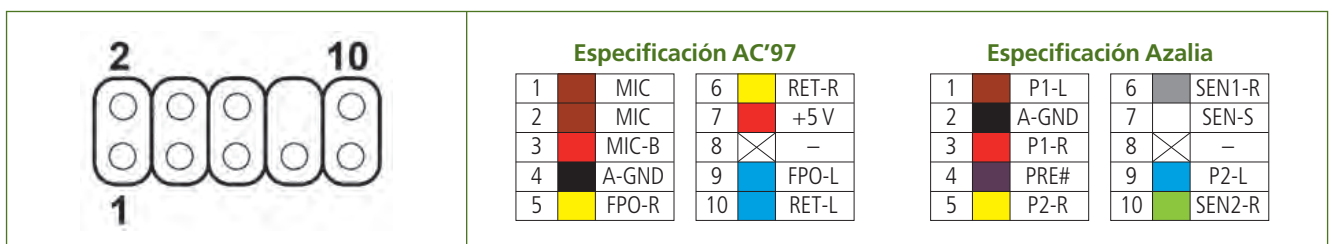
↑ Cabecera de audio frontal Azalia.
