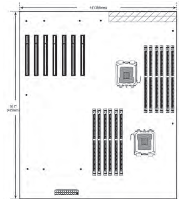
↑ Esquema del factor de forma WTX.
