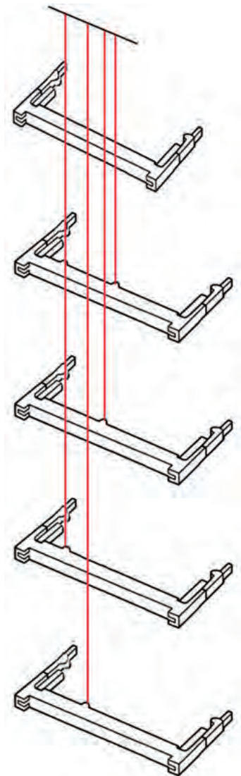
↑ Ubicación de las guías en los zócalos SO-DIMM (de arriba abajo: 72, 100, 144, 200 y 204 contactos).
