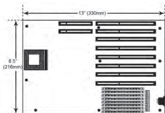
↑ Esquema del factor de forma Baby-AT.
