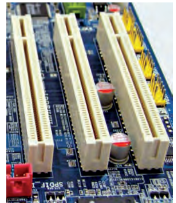
↑ Slots PCI de 32 bits a 3,3 V.
