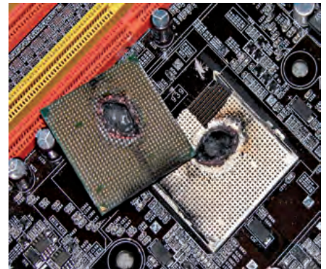
↑ Microprocesador y socket quemados por sobrecalentamiento.
