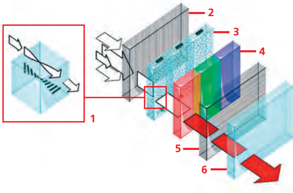
↑ Partes principales de un monitor LCD:
