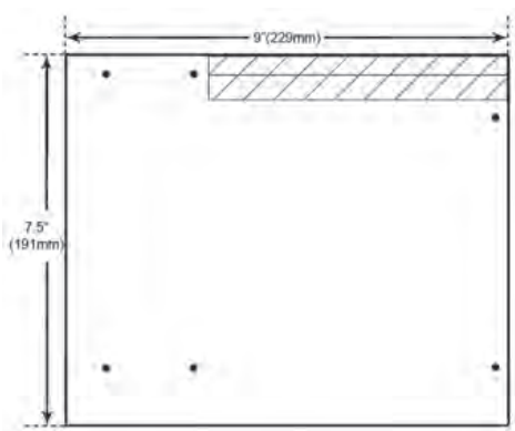
↑ Esquema del factor de forma Flex-ATX.
