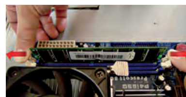
↑ Extracción del módulo de memoria.
