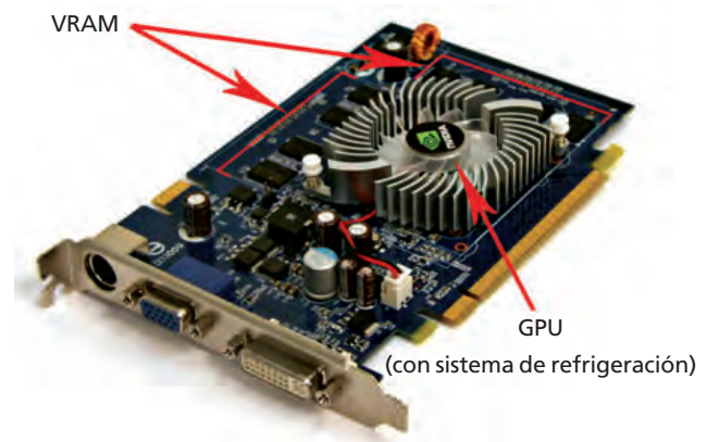
↑ Tarjeta gráfica.
