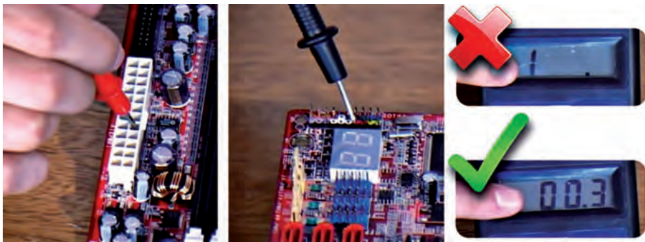
↑ Uno de los polos va al pin 14 del ATX.
