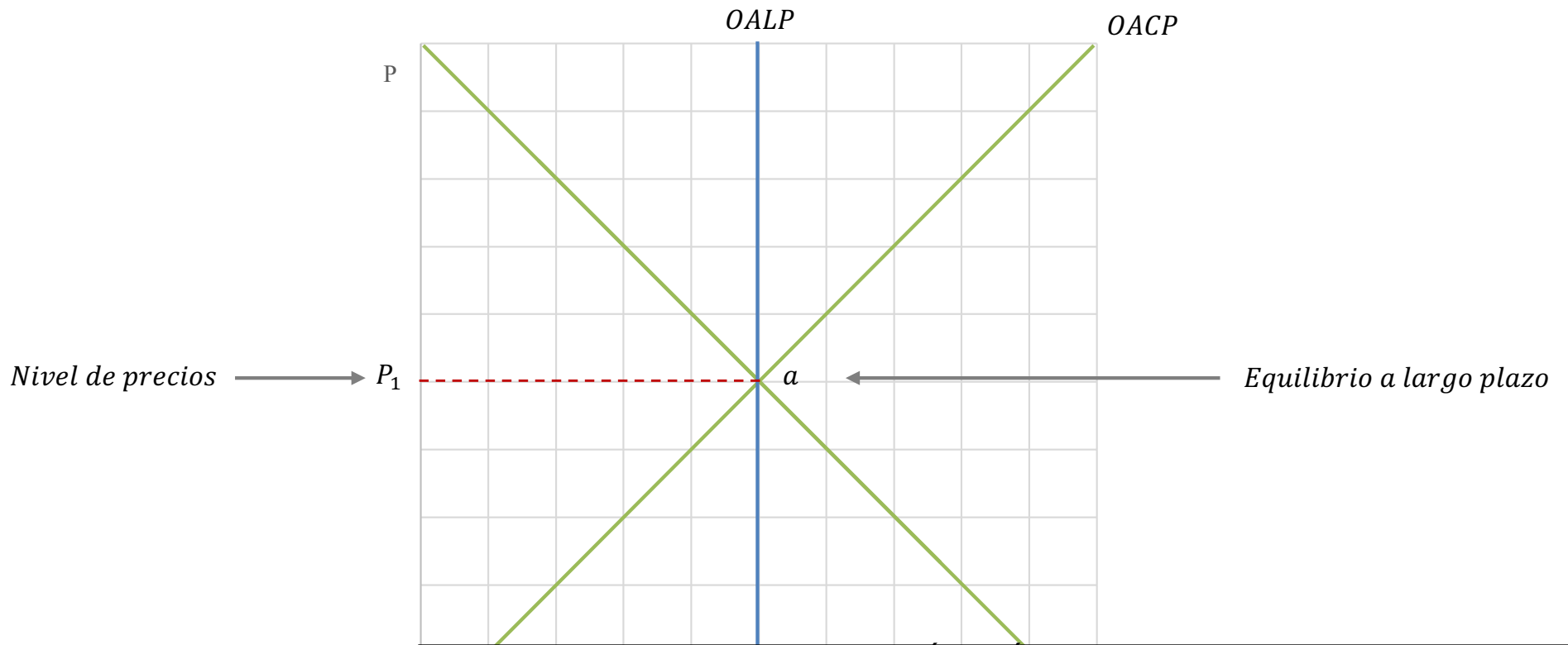
Figura 12.17. Equilibrio macroeconómico
