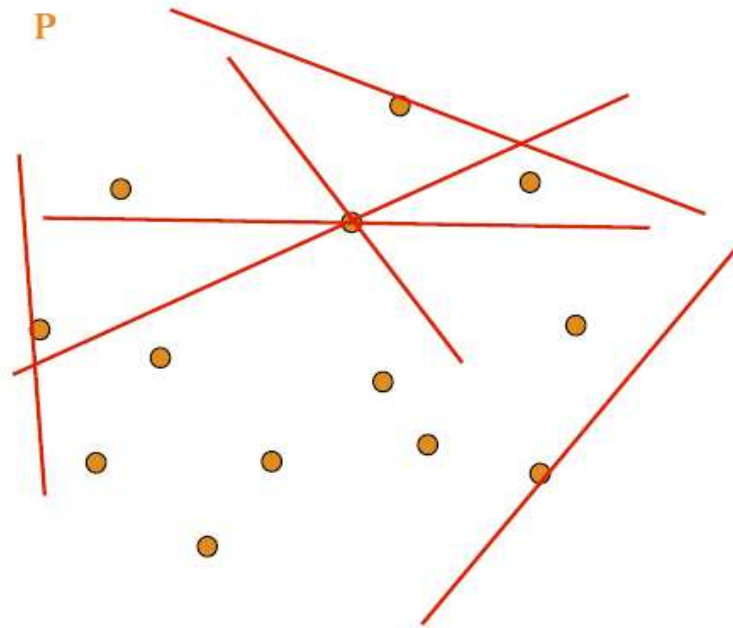
Imagen 3.4. Ejemplo ilustrativo de la tercera propiedad.
