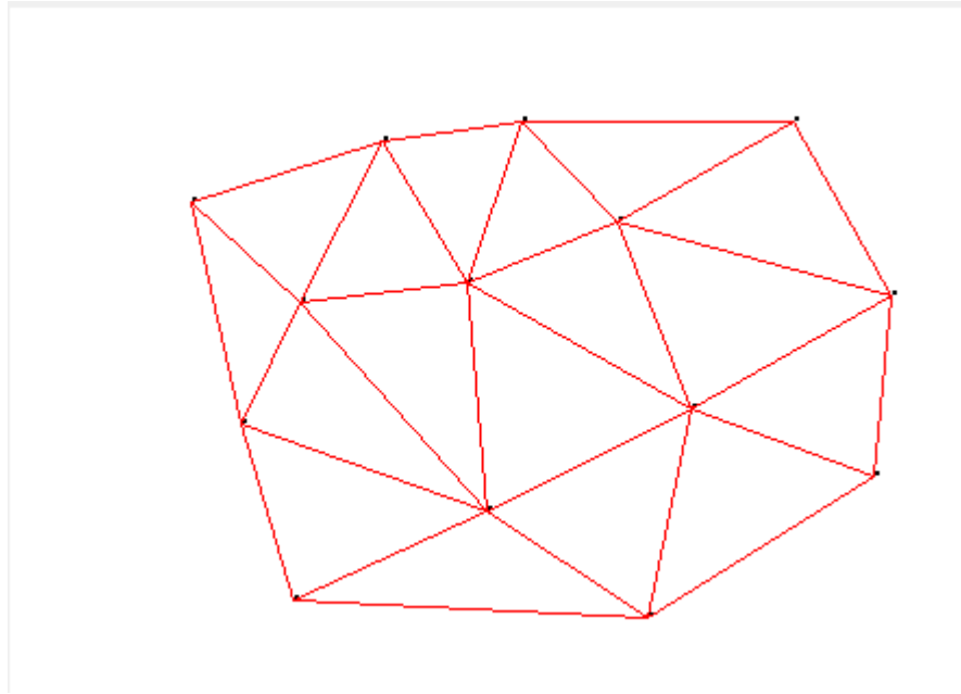
Imagen 3.7. Triangulación de Delaunay de la nube de puntos de la figura 3.6.
