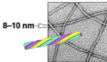
Filamentos intermedios
