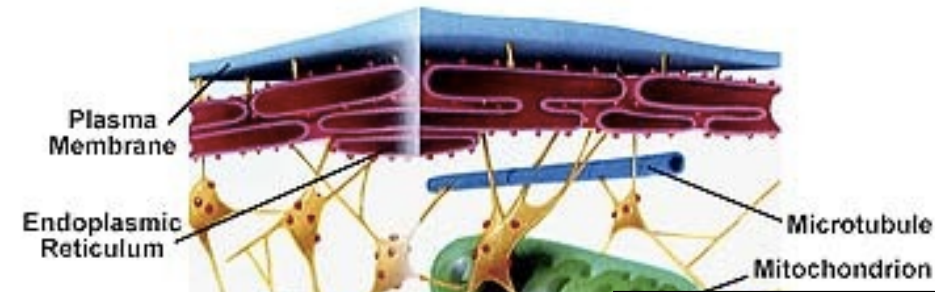
Filamentos intermedios
