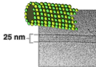
Microtúbulos
