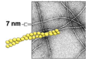
Microfilamentos
