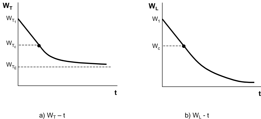
Figura 3. Condiciones de secado constantes: curvas de secado
