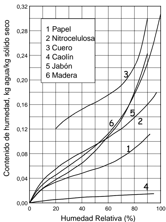
Figura 1. Curvas de equilibrio a 25°C para diferentes materiales
