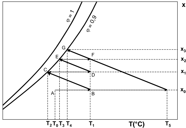
Figura 7. Condiciones del aire mediante secado con calefacción inicial del aire solamente o con recirculación repetida del mismo.
