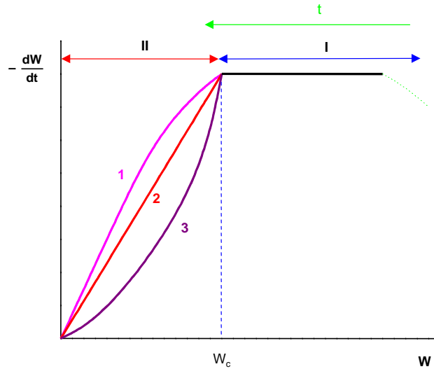
Figura 4. Condiciones de secado constantes: curvas de velocidad de secado características
