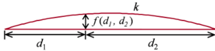
FIGURA 20.15: CORRECCIÓN DE LA ALTURA DEL PERFIL DEL VANO MEDIANTE EL MÉTODO FLECHA.
