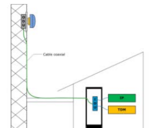
FIGURA 13.2: INSTALACIÓN SPLIT-MOUNT.
