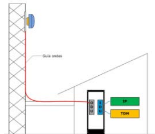
FIGURA 13.1: INSTALACIÓN FULL-INDOOR.
