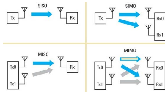
FIGURA 29.1: TIPOS DE SISTEMAS QUE APLICAN DIVERSIDAD ESPACIAL.
