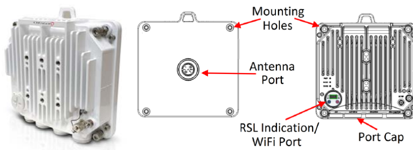
FIGURA 2.3: IP20-E, ODU FULL-INDOOR PARA LA BANDA E DEL FABRICANTE CERAGON.
