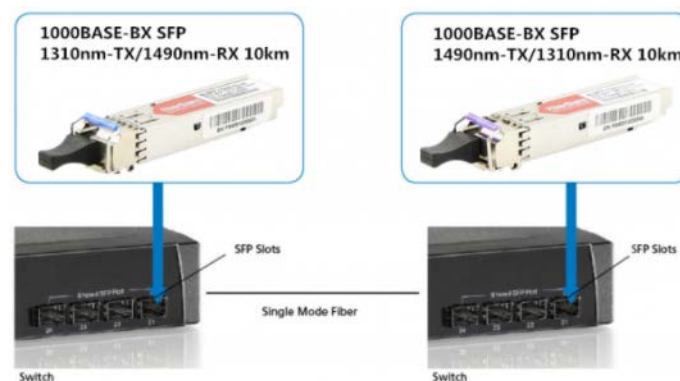
FIGURA 12.17: CONEXIÓN ENTRE TRANSCEIVERS SFP BiDi.
