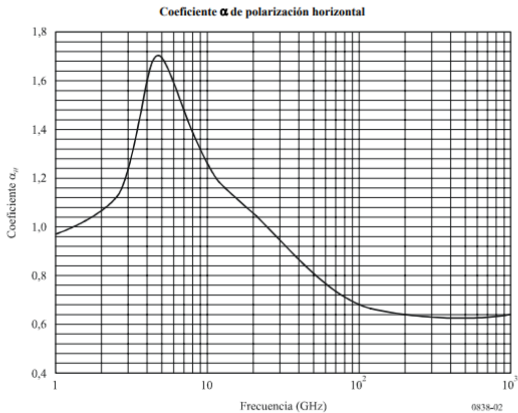
FIGURA 22.4: VALOR DE \alpha EN FUNCIÓN DE LA FRECUENCIA PARA POLARIZACIÓN HORIZONTAL.
