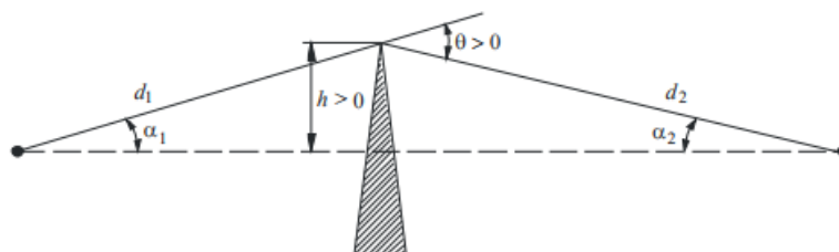
FIGURA 20.10: PARÁMETRO GEÓMETRICOS EN ESCENARIO NON LINE OF SIGHT CON ÚNICO OBSTÁCULO EN ARISTA EN FILO DE CUCHILLO.
