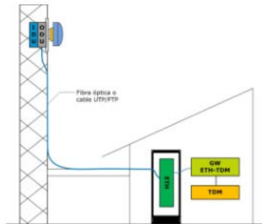
FIGURA 13.3: INSTALACIÓN FULL-OUTDOOR.
