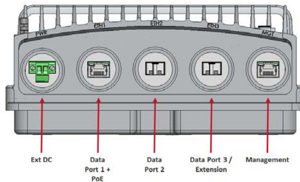
FIGURA 5.13: PUERTOS DE LAS ODU S IP20-S E IP20-C.
