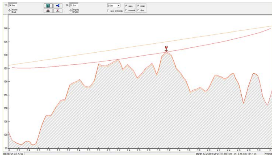
FIGURA 20.13: HERRAMIENTA DE DISEÑO PATHLOSS, MOSTRANDO EL PERFIL DEL VANO TENIENDO EN CUENTA LA CURVATURA TERRESTRE, LA LÍNEA DE VISIÓN DIRECTA, LA PRIMERA ZONA DE FRESNEL Y CALCULA LA ALTURA DE LAS ANTENAS PARA UN ESCENARIO LOS.
