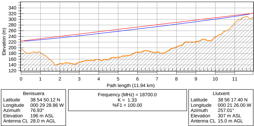
FIGURA 5.20: PERFIL DEL VANO BENISSUERA - LLUTXENT.
