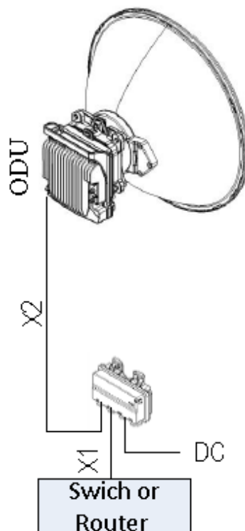
FIGURA 12.15: LIMITACIONES EN LA LONGITUD DE LOS CABLES DEBIDO AL USO DE PoE.
