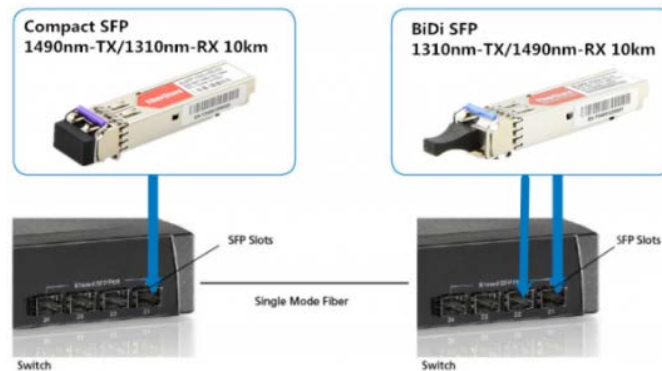
FIGURA 12.18: CONEXIÓN ENTRE TRANSCEIVERS CSFP Y SFP BIDI.
