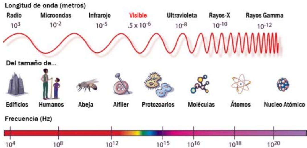
FIGURA 2.1: ESPECTRO ELECTROMAGNÉTICO.
