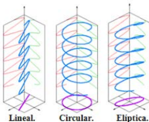
FIGURA 17.2: FORMA DISEÑADA POR EL VECTOR CAMPO ELÉCTRICO EN LA PROPAGACIÓN DE ONDA ELECTROMAGNÉTICA.
