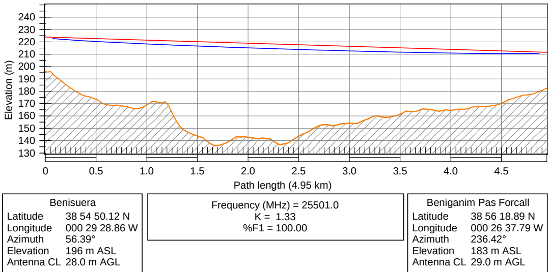
FIGURA 5.18: PERFIL DEL VANO BENISSUERA – BENIGÀNIM PAS FORCALL.
