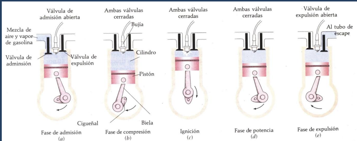
Figura 17-3 Motor de combustión interna. En (a), cuando el pistón desciende entra en la cámara de combustión una mezcla de aire y vapor de gasolina. El pistón entonces asciende en (b), comprimiendo el gas para su ignición en (c).
