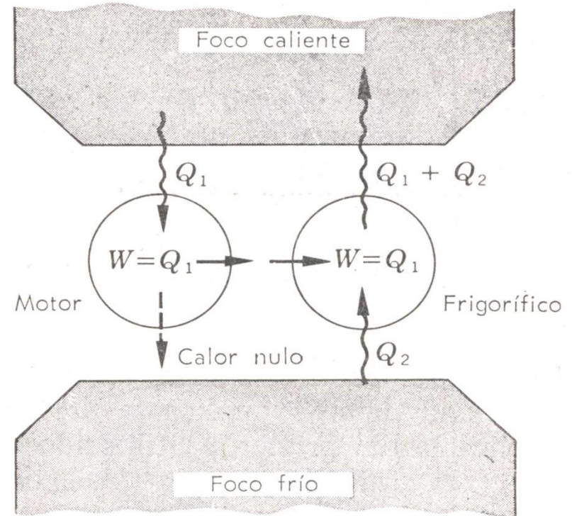
FIG. 7-11. Demostración de que -K \supset -C .
