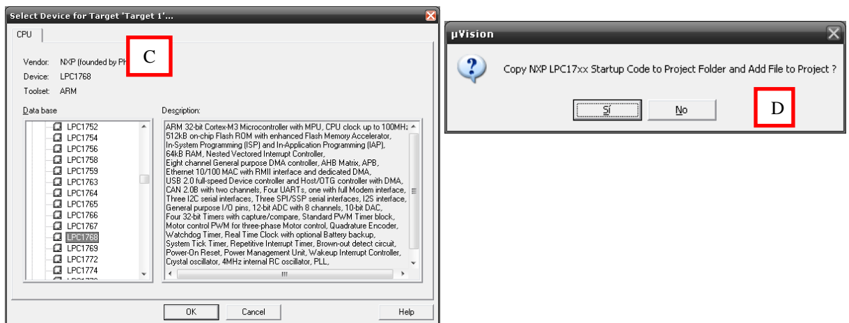
Figura 3. Ventanas para crear un nuevo proyecto, seleccionar el fabricante y el dispositivo.
