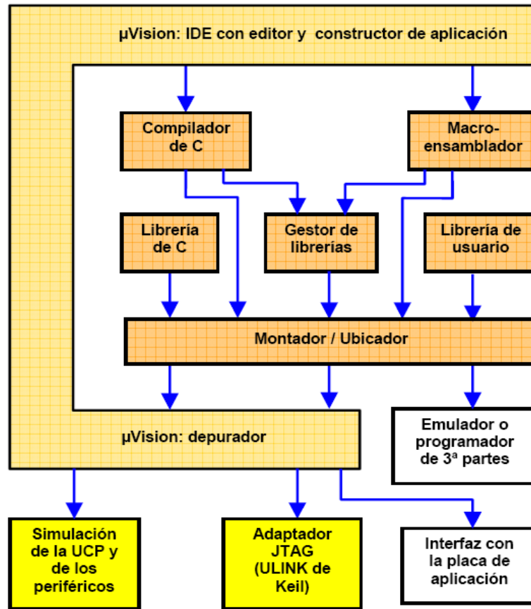
Figura 1. Componentes del entorno de desarrollo Keil µVision®.
