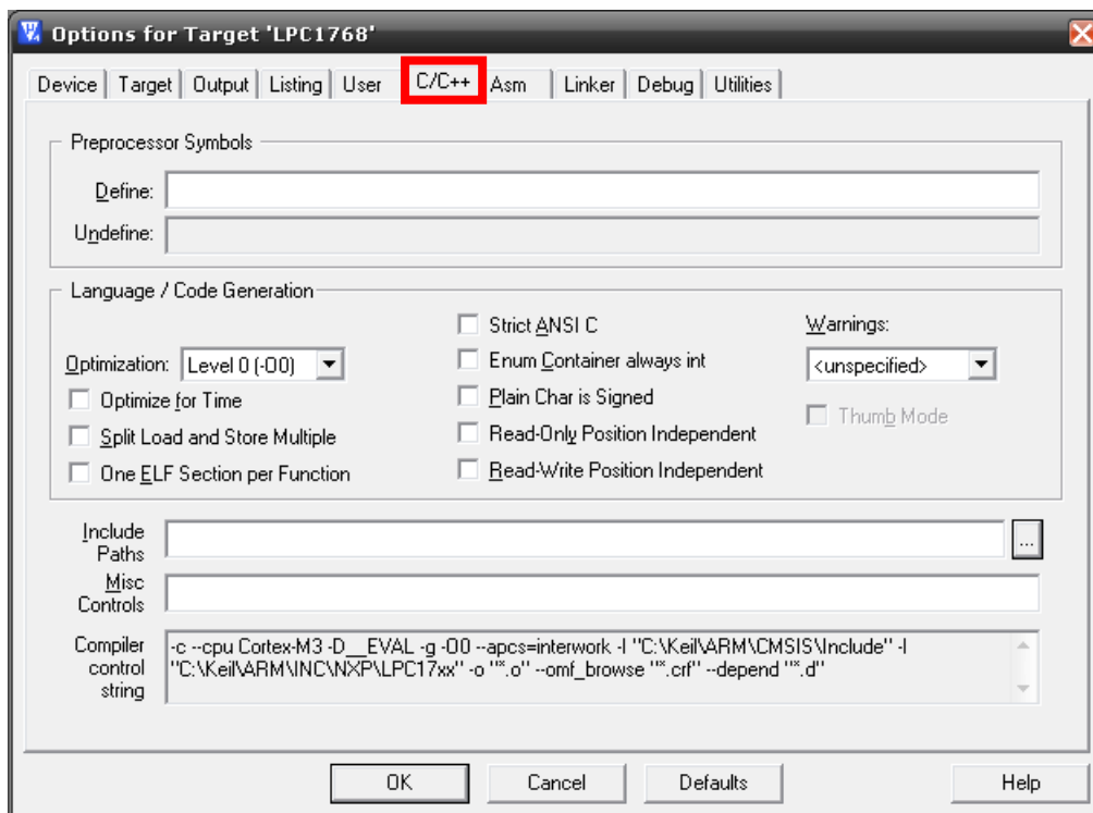
Figura 6C. Opciones para la pestaña C/C++.
