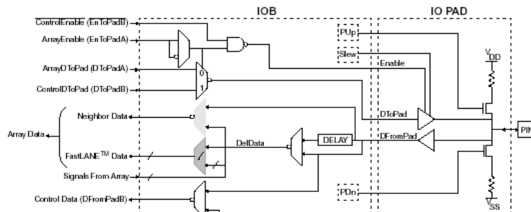
Diagrama de bloques de la celda de E/S de la XC6200
