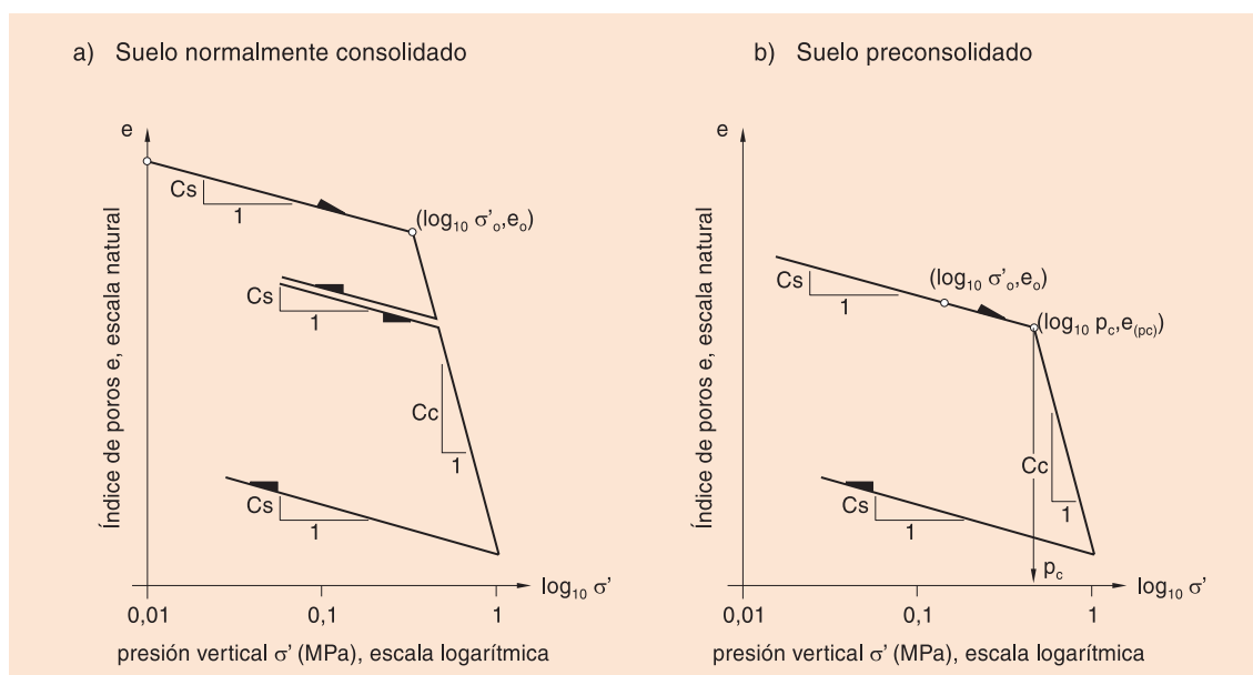
FIGURA 4.12. ENSAYO EDMÉTRICO. PARÁMETROS BÁSICOS DE CÁLCULO
