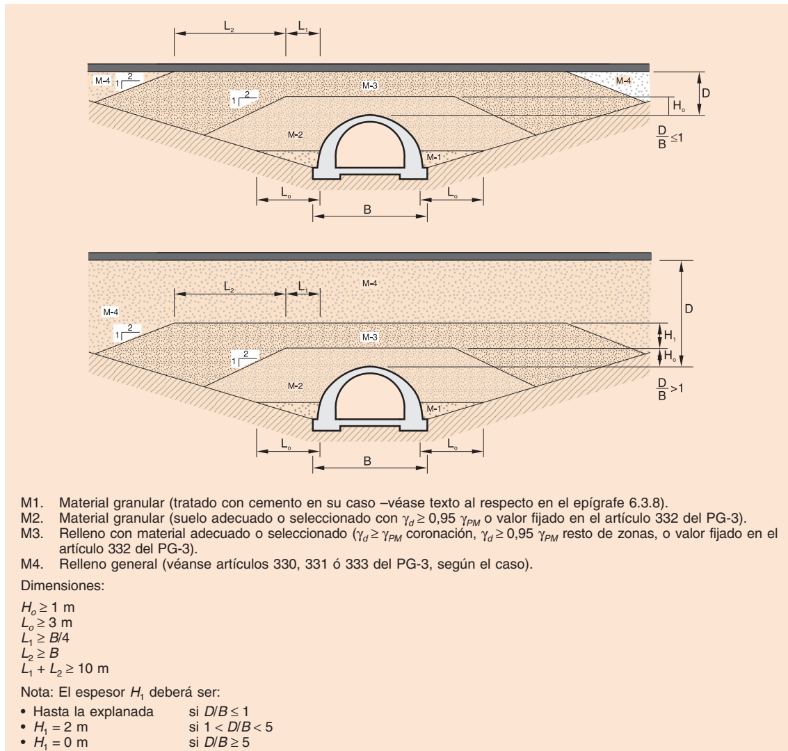
FIGURA 6.14. EJEMPLOS DE CUÑAS DE TRANSICIÓN EN UNA ESTRUCTURA ENTERRADA
