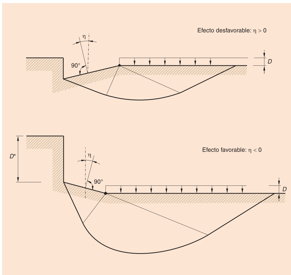
FIGURA 4.8. CIMENTACIONES SOBRE PLANOS NO HORIZONTALES
