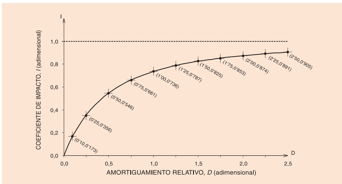
FIGURA 5.9. COEFICIENTE DE IMPACTO I , EN FUNCIÓN DEL AMORTIGUAMIENTO RELATIVO D
