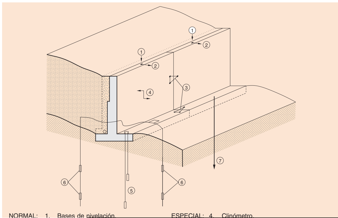
FIGURA 8.2. ESQUEMA DE POSIBLE AUSCULTACIÓN DE UN ESTRIBO DE PUENTE
