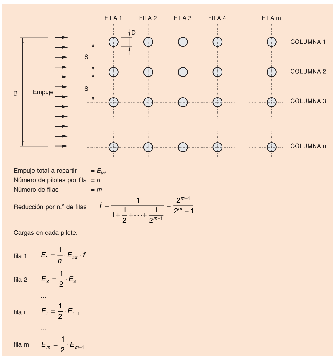
FIGURA 5.6. EFECTO GRUPO EN LOS ESFUERZOS PARÁSITOS HORIZONTALES
