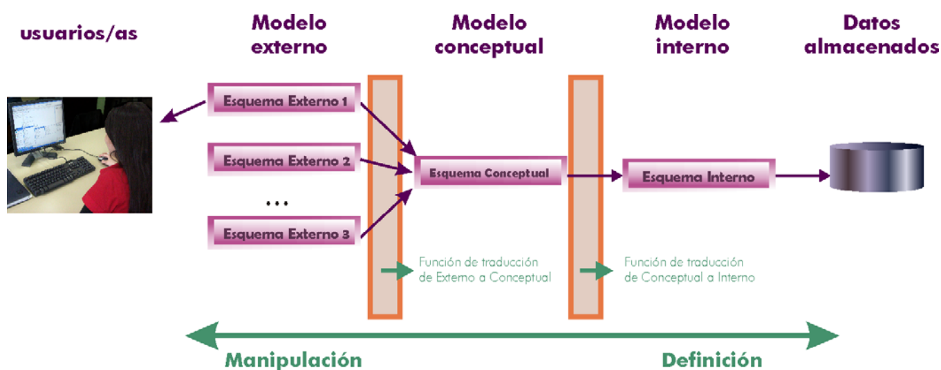
Ilustración 7, Niveles en el modelo ANSI
